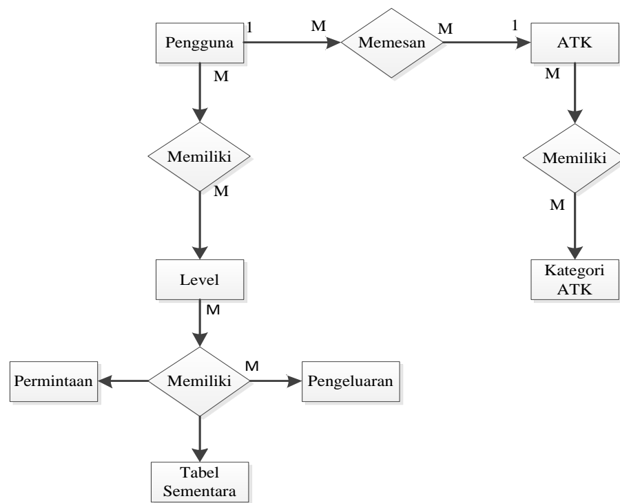
Gambar IV. 9. ERD
