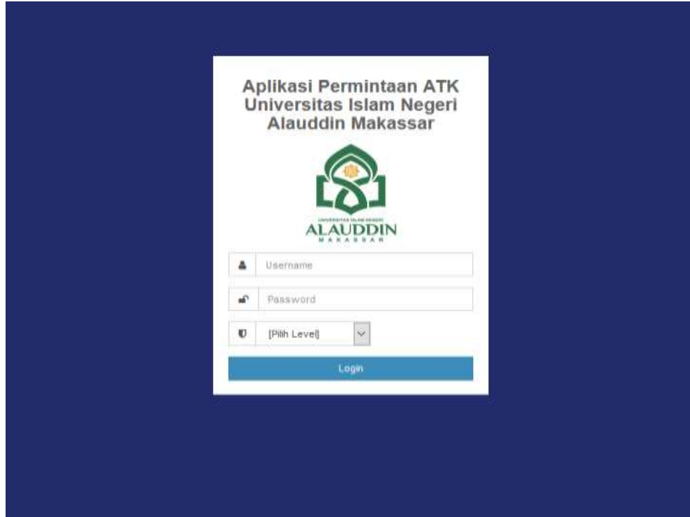
Gambar V. 1. Antarmuka Login
