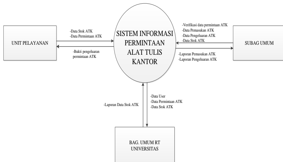
Gambar IV. 4. Diagram Konteks
