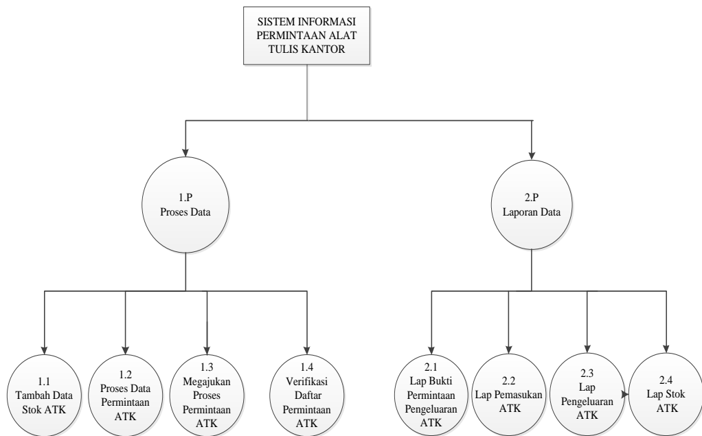
Gambar IV. 3. Diagram Berjenjang
