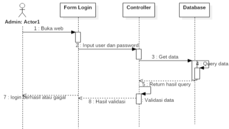
Gambar IV.5 Sequence Diagram untuk Login Admin
