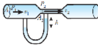
Gambar. Venturimeter dengan manometer
