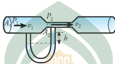
Gambar. Venturimeter dengan manometer
