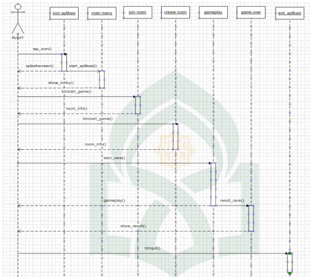
Gambar IV.11 Sequence Diagram sistem yang akan dibuat
