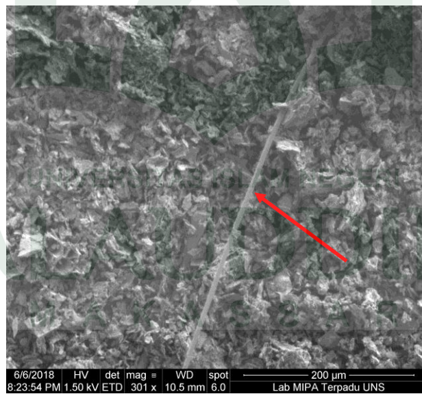
Gambar 4.7 Morfologi SEM CNT Karbon Aktif dengan Katalis perbesaran 301 X
