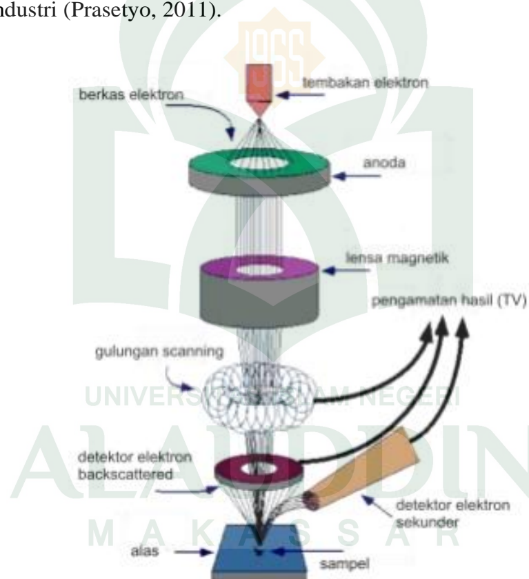
Gambar 2.12 Skema prinsip kerja SEM
