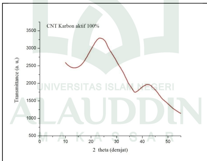
Grafik 4.5 Pola Fasa Difraksi CNT Karbon Aktif 100% Puncak tertinggi pada 2\theta = 24,97^{\circ} , dan puncak lainnya 2\theta = 43,27^{\circ}
