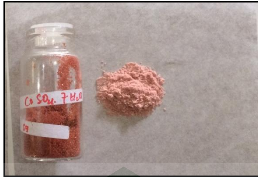
Gambar 2.9 katalis \text{CoSO}_4
