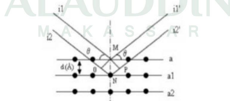
Gambar 2.11 Difraksi sinar x atom pada bidang
