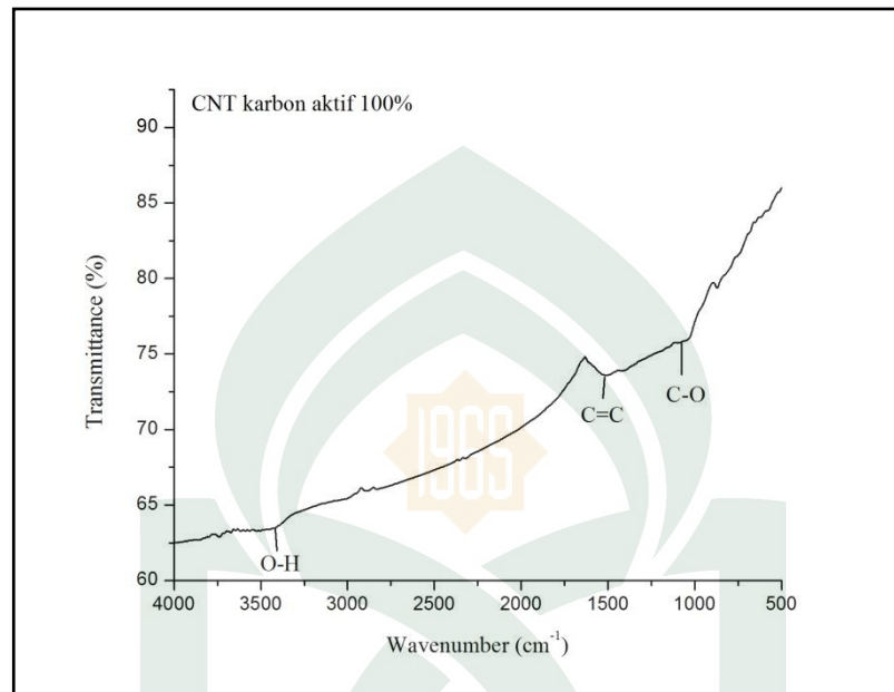
Grafik 4.3 Grafik FTIR CNT Karbon Aktif
