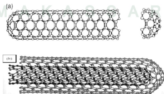
Gambar 2.7 Struktur Carbon nanotubes , a) struktur SWNT, b) struktur MWNT
