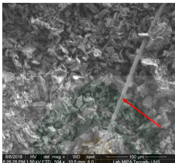
Gambar 4.8 Morfologi SEM CNT Karbon Aktif dengan Katalis perbesaran 504 X
