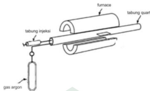
Gambar 2.8 Metode CVD
