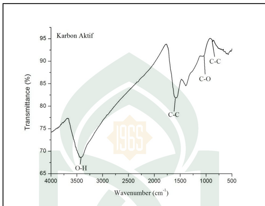
Grafik 4.1 Grafik FTIR Karbon Aktif
