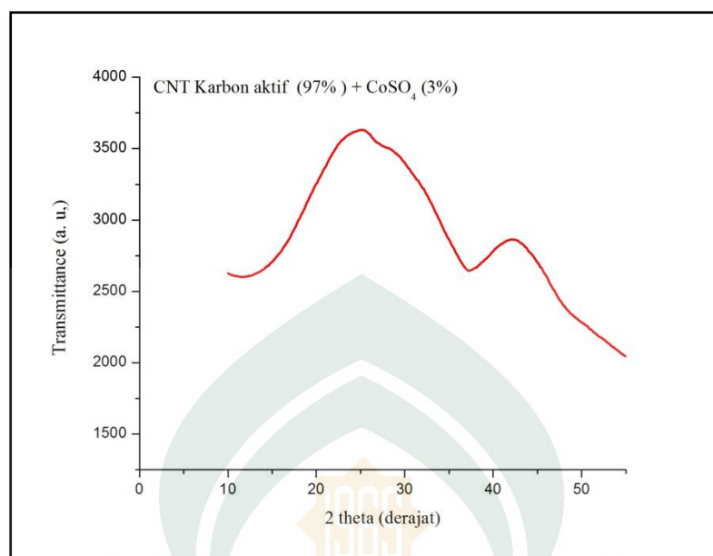
Grafik 4.6 Pola Fasa Difraksi CNT Karbon Aktif dengan Katalis CoSO 4 Puncak tertinggi pada 2\theta = 24,75^\circ , dan puncak lainnya 2\theta = 43,75^\circ
