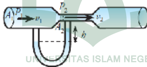
Gambar. Venturimeter dengan manometer
