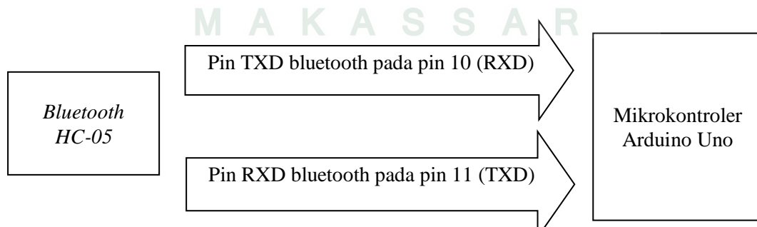
Gambar IV.5 Ilustrasi Bluetooth pada masing masing mikrokontroler
