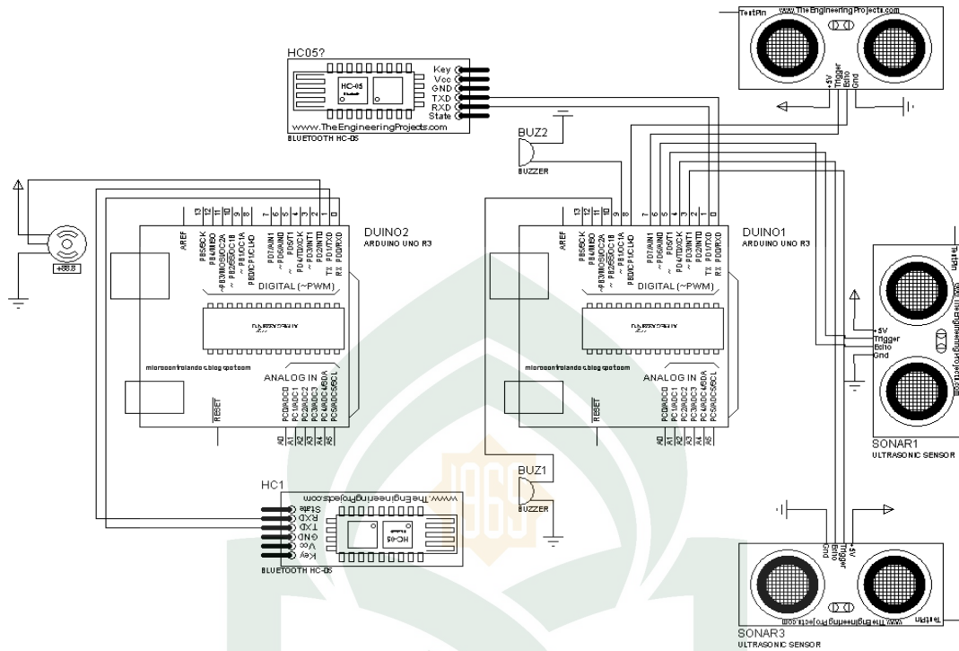
Gambar IV.3 Rancangan Desain Keseluruhan Alat
