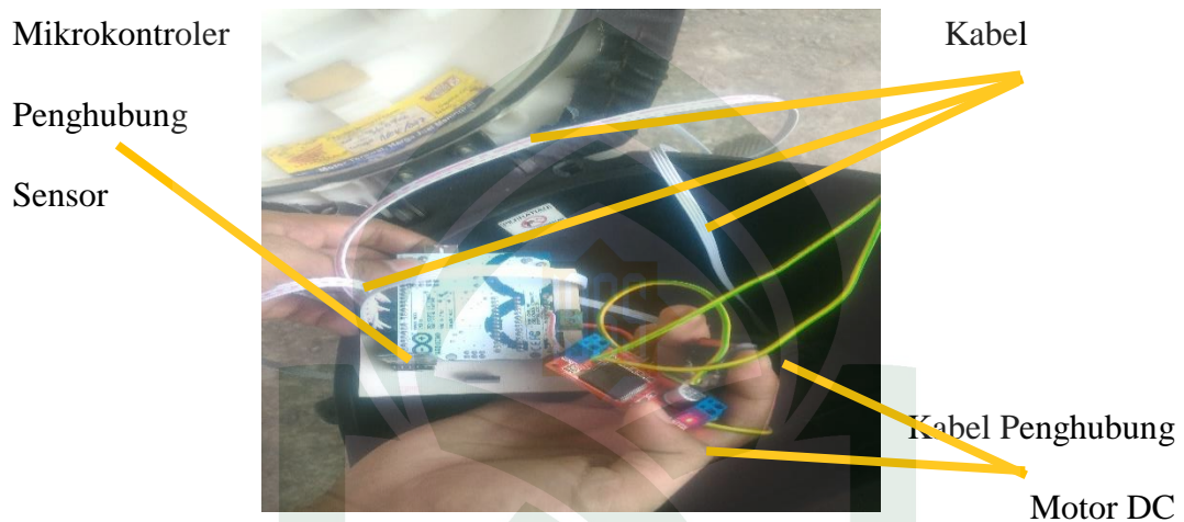
Gambar V.9 Pemasangan Mikrokontroler Arduino Uno dan Kabel Penghubung antar Komponen
