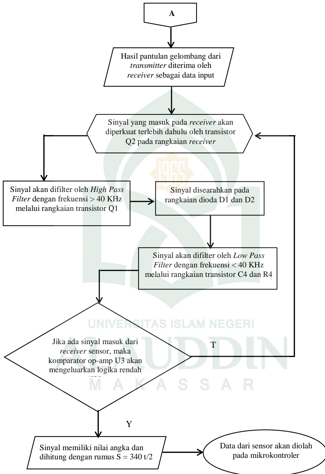
Gambar IV.9 Flowchart tentang proses scanning pada sensor ultrasonik
