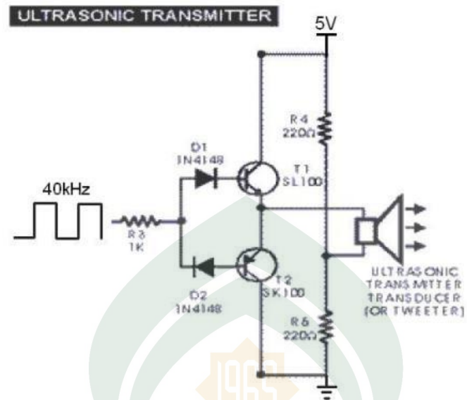
Gambar IV.10 Gambar rangkaian Transmitter pada sensor ultrasonik
