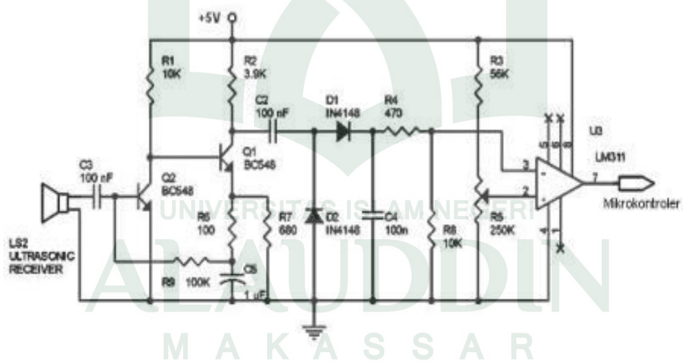
Gambar IV.11 Gambar rangkaian Receiver pada sensor ultrasonik
