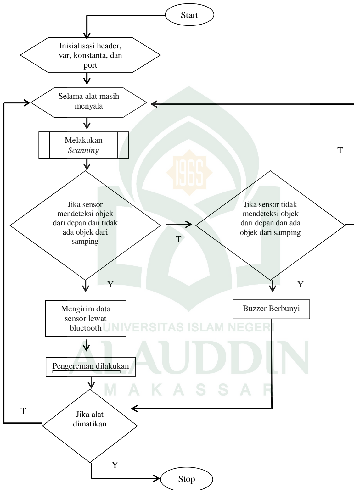
Gambar IV.8 Flowchart Sistem Pengereman Otomatis Dan Blindspot Warning
