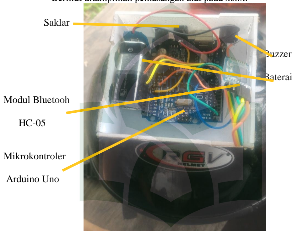
Gambar V.6 Pemasangan Alat pada Helm
