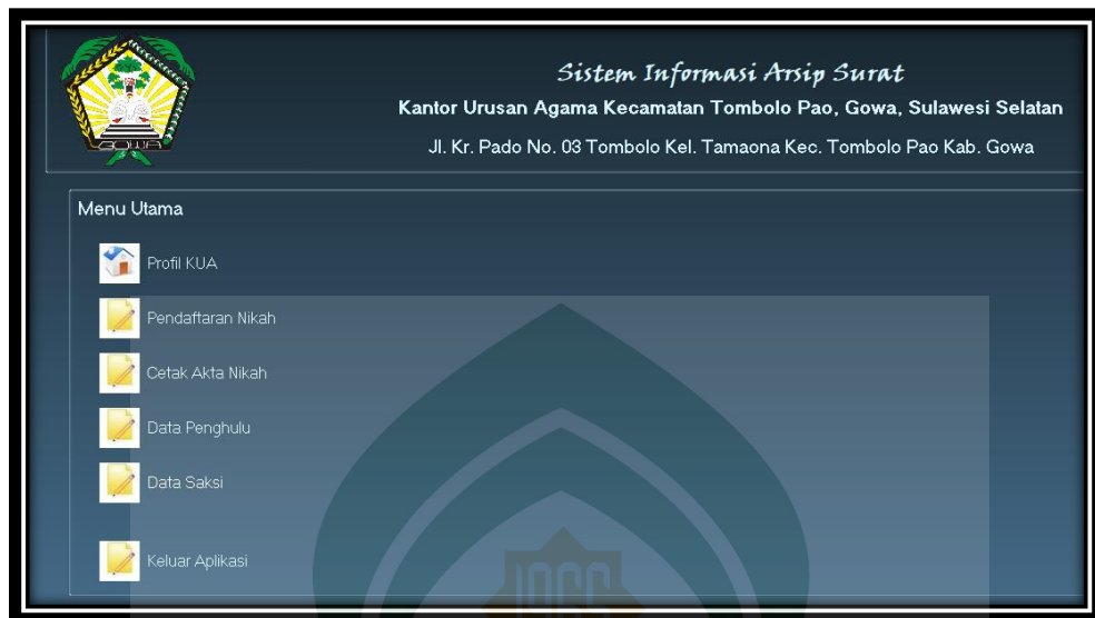
Gambar V.2 Menu Utama
