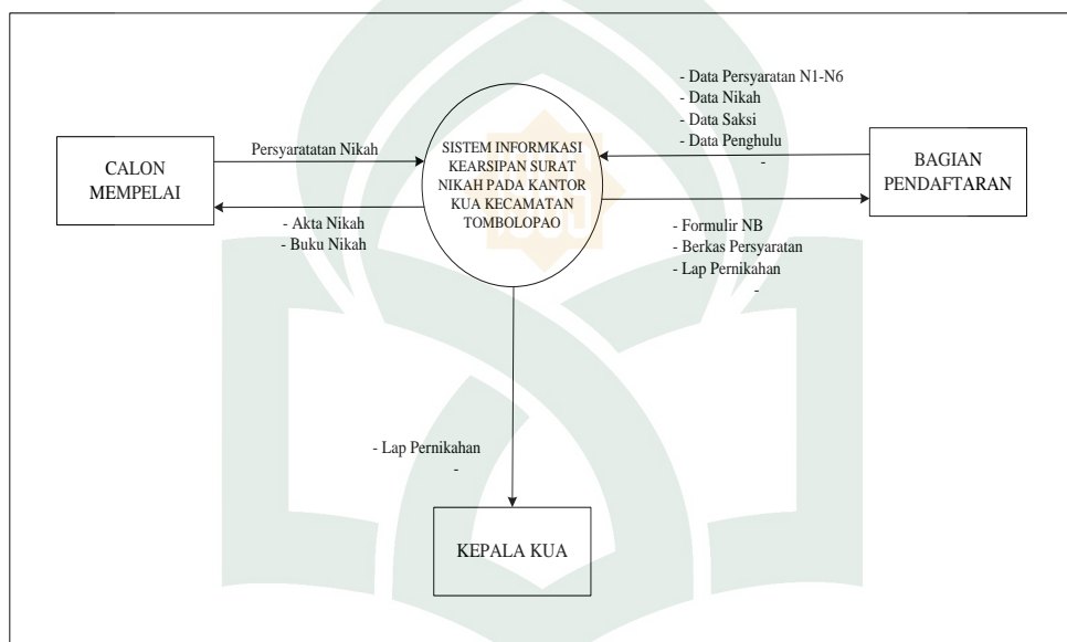
Gambar IV.3 Diagram Konteks
