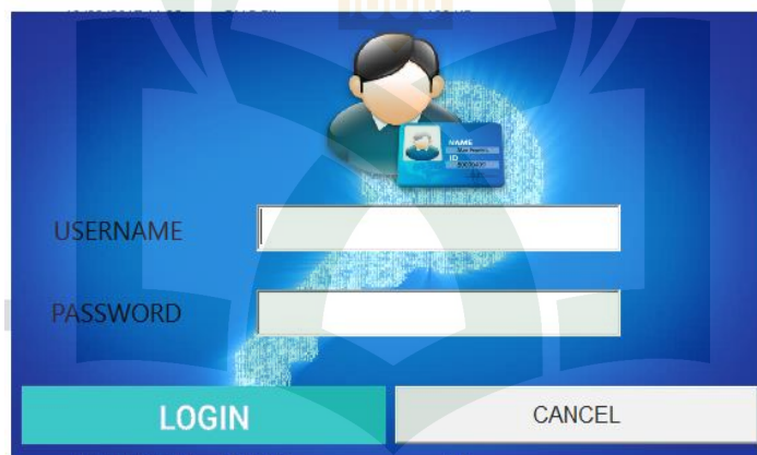
Gambar V.1 Halaman Login
