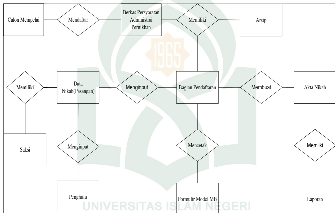
Gambar IV.9 ERD
