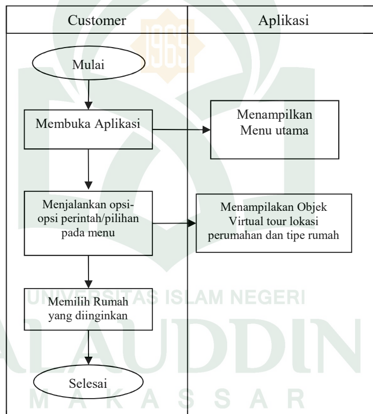
Gambar IV.2 Flowmap diagram yang diusulka
