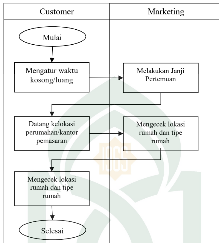
Gambar IV.1 Flowmap sistem yang berjalan
