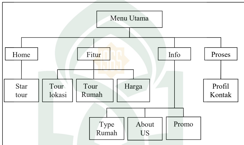
Gambar IV.10 Struktur Navigasi
