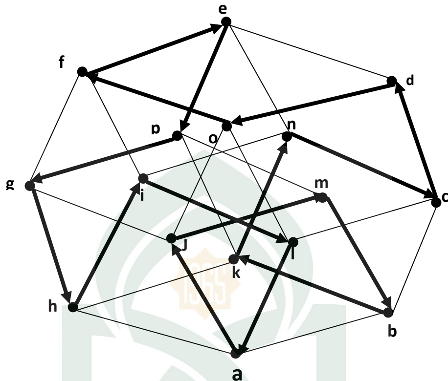
Gambar 4.11 Lintasan Hamilton dari Graf Kubus Q_4 .
