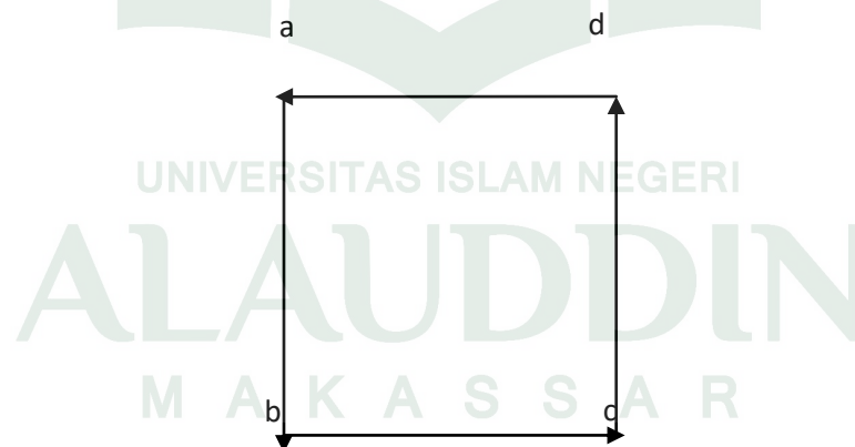
Gambar 2.11. Graf Hamilton
