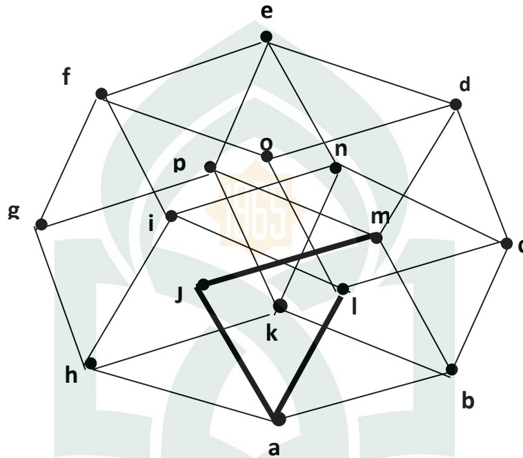
Gambar 4.9 Langkah 2 dalam Menentukan lintasan Hamilton pada Graf Kubus Q_4 .
