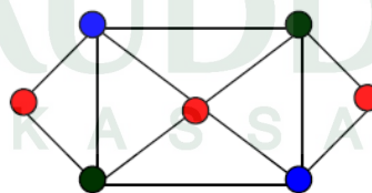
Gambar 2.16. Pewarnaan Graf
