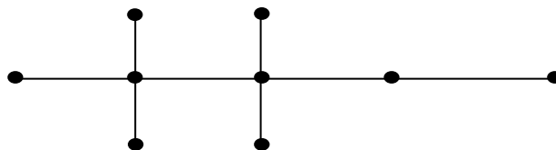
Gambar 2.9. Graf Pohon
