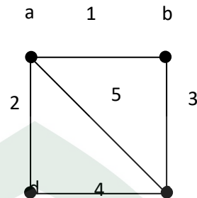
Gambar 2.4. Lintasan pada Graf G
