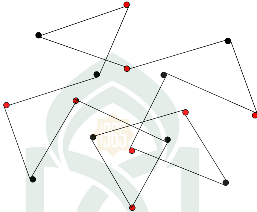
Gambar 4.13 Pewarnaan Titik pada Backbone Lintasan Hamilton.
