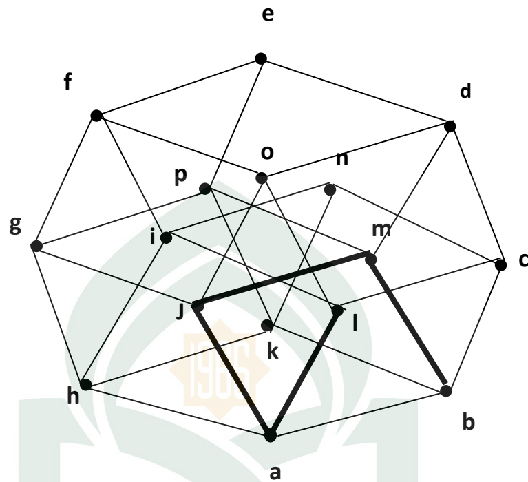
Gambar 4.10 Langkah 3 dalam Menentukan lintasan Hamilton pada Graf Kubus Q_4 .
