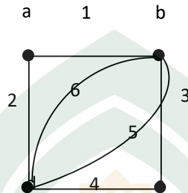
Gambar 2.6. Sirkuit pada Graf G
