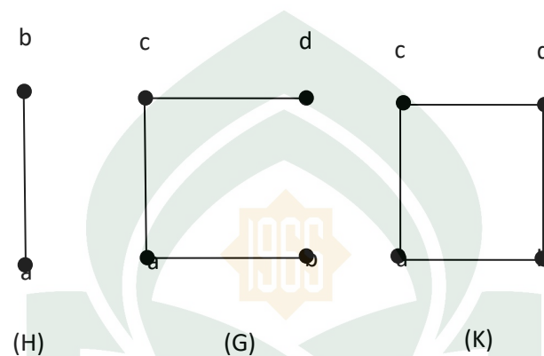
Gambar 2.14. Subgraf
