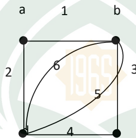
Gambar 2.3. Jalan pada Graf G
