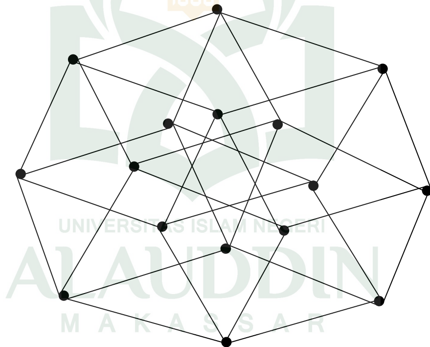
Gambar 4.1 Graf kubus Q_4 .
