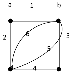
Gambar 2.7. Sikel pada Graf G
