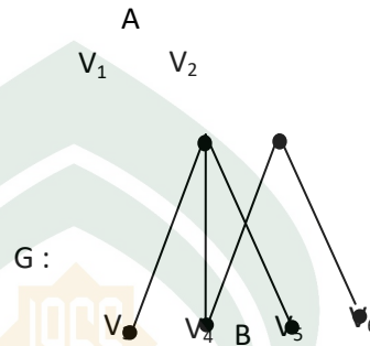
Gambar 2.12. Graf bipartisi
