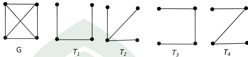
Gambar 2.20. Backbone Pohon
