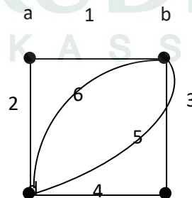
Gambar 2.5. Jejak pada Graf G
