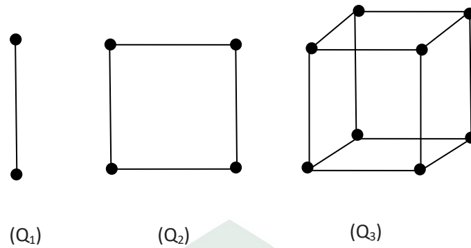
Gambar 2.15. Graf kubus
