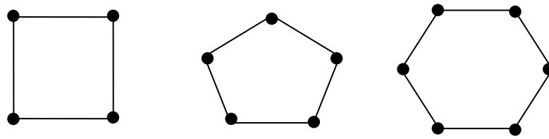
Gambar 2.8. Graf planar
