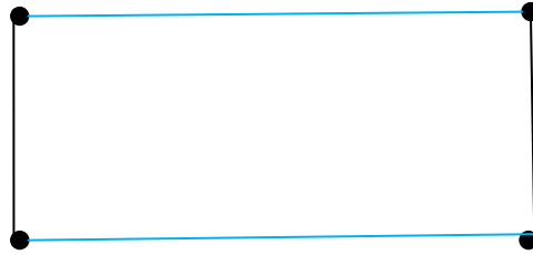
Gambar 2.18. Pewarnaan Sisi
