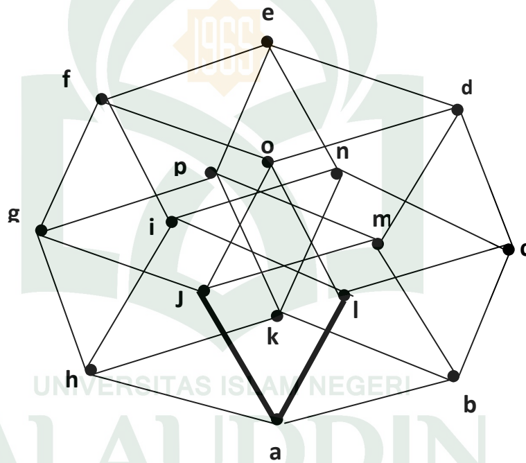
Gambar 4.8 Langkah 1 dalam Menentukan lintasan Hamilton pada Graf Kubus Q_4 .
