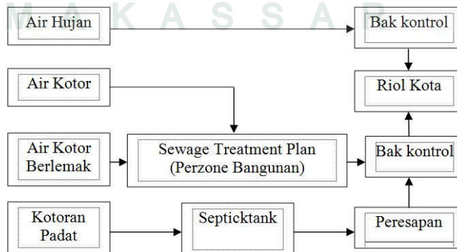
Gambar 70. Pengolahan air Kotor (Sistem bangunan pintar;2006)
