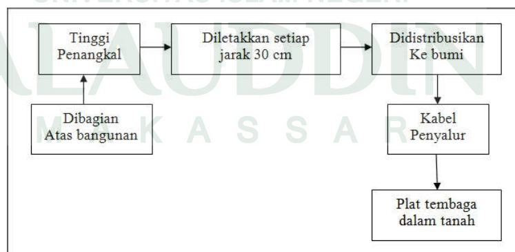
Gambar 76. Sistem Penangkal petir (Sistem bangunan pintar;2006)
