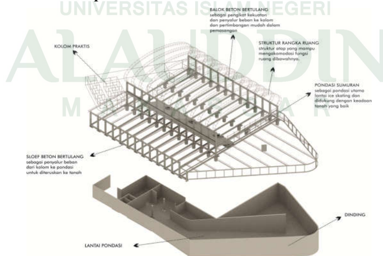
Gambar 84. Konsep Struktur Bangunan Utama (Olah data;2017)
