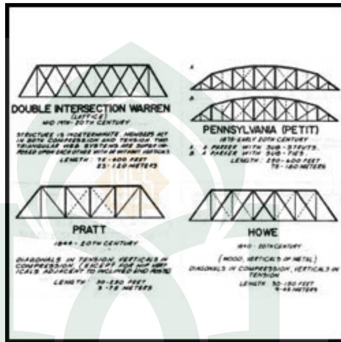
Gambar 24 : Prinsip distribusi gaya Sumber : Wurm, 2007
