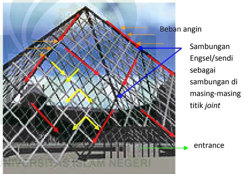
Gambar 23 : Diagram distribusi gaya pembebanan museum Louvre Sumber : Wurm, 2007
