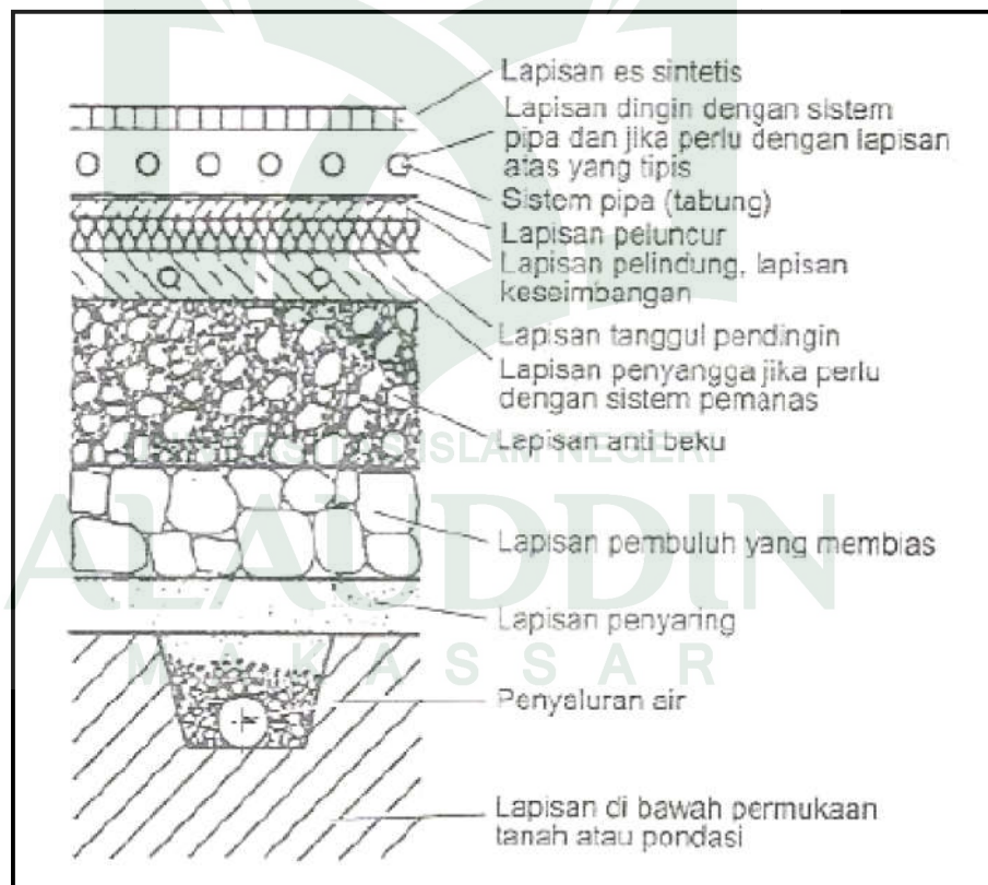
Gambar 3 : Detail lapisan lantai arena seluncur es
