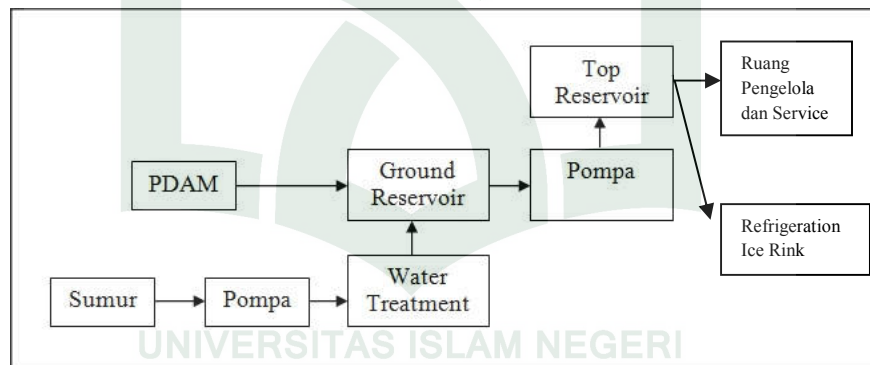
Gambar 69. Skema distribusi air bersih (Sistem bangunan pintar;2006)
