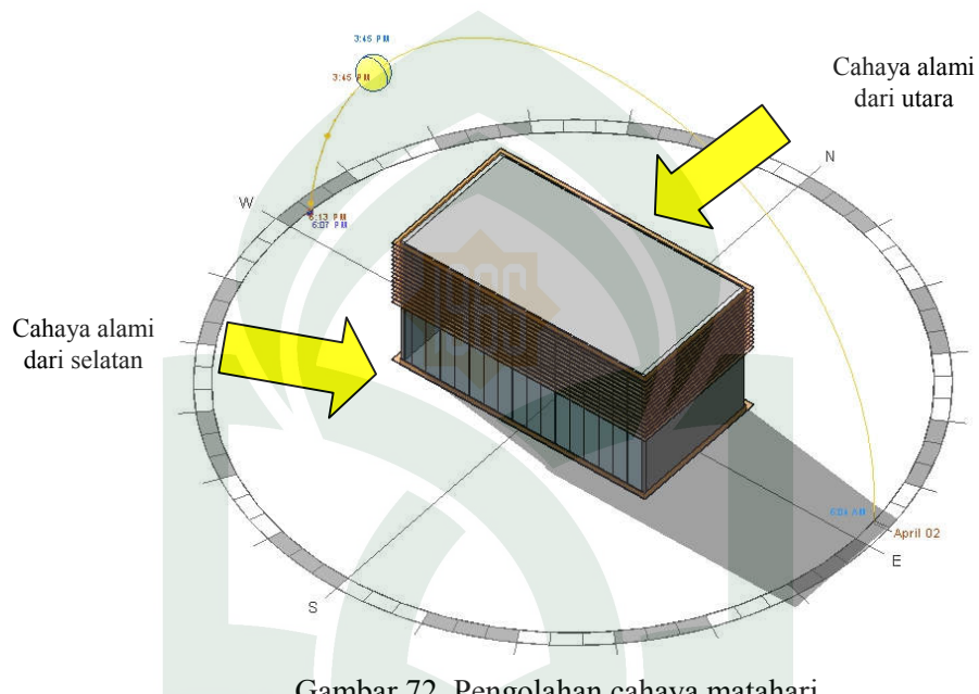
Gambar 72. Pengolahan cahaya matahari (Analisis pribadi, 2014)
