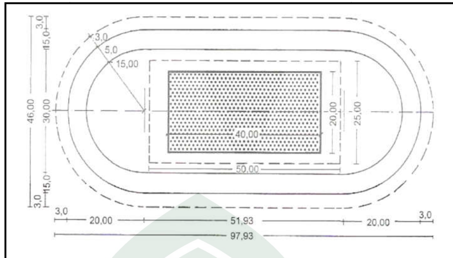
Gambar 1 : Lintasan arena seluncur es 20 x 40 Sumber : Data Arsitek Jilid 1 , Edisi 2 (1996:22)
