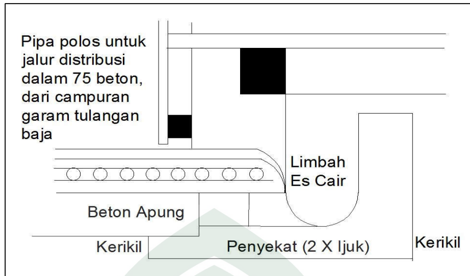
Gambar 4 : Detail pipa tanam Sumber : Data Arsitek Jilid 1, Edisi 2, hal.26
