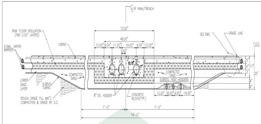
Gambar 55. Potongan bantalan parit lantai seluncur es Sumber : IIHF Ice Rink Guide
