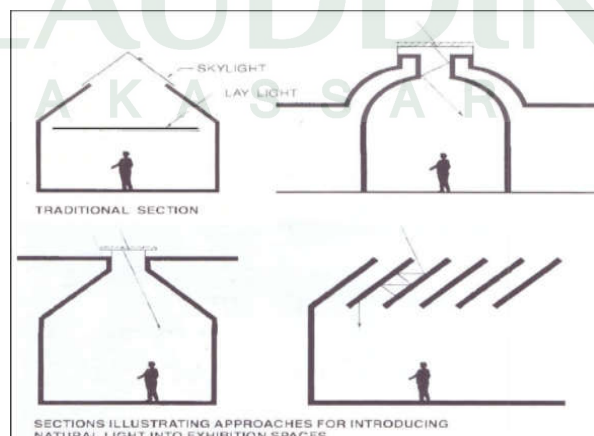
Gambar 73. Teknik pencahayaan alami (Time saver standard, )
