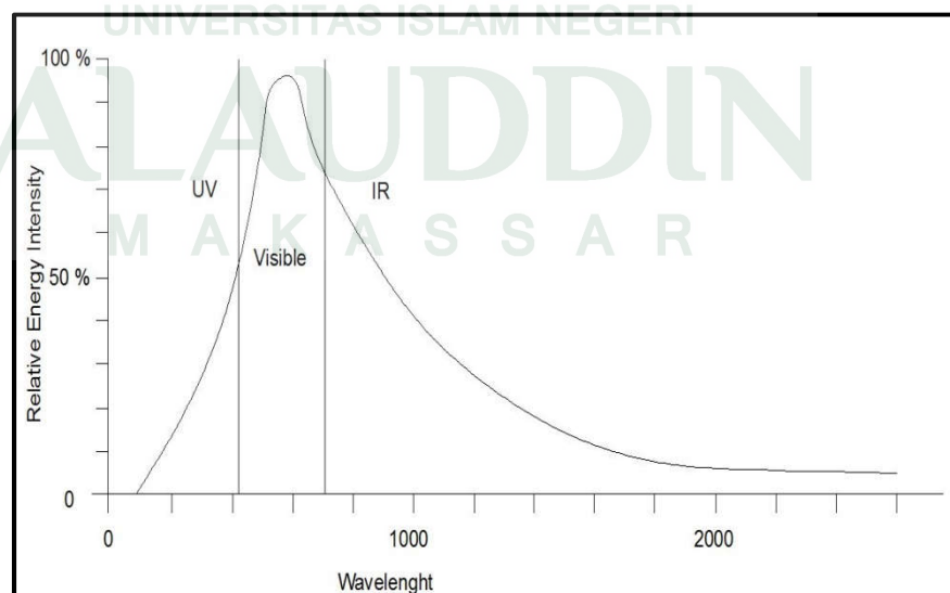
Gambar 13 : Spektrum cahaya matahari yang jatuh pada kaca Sumber : Wurm, 2007
