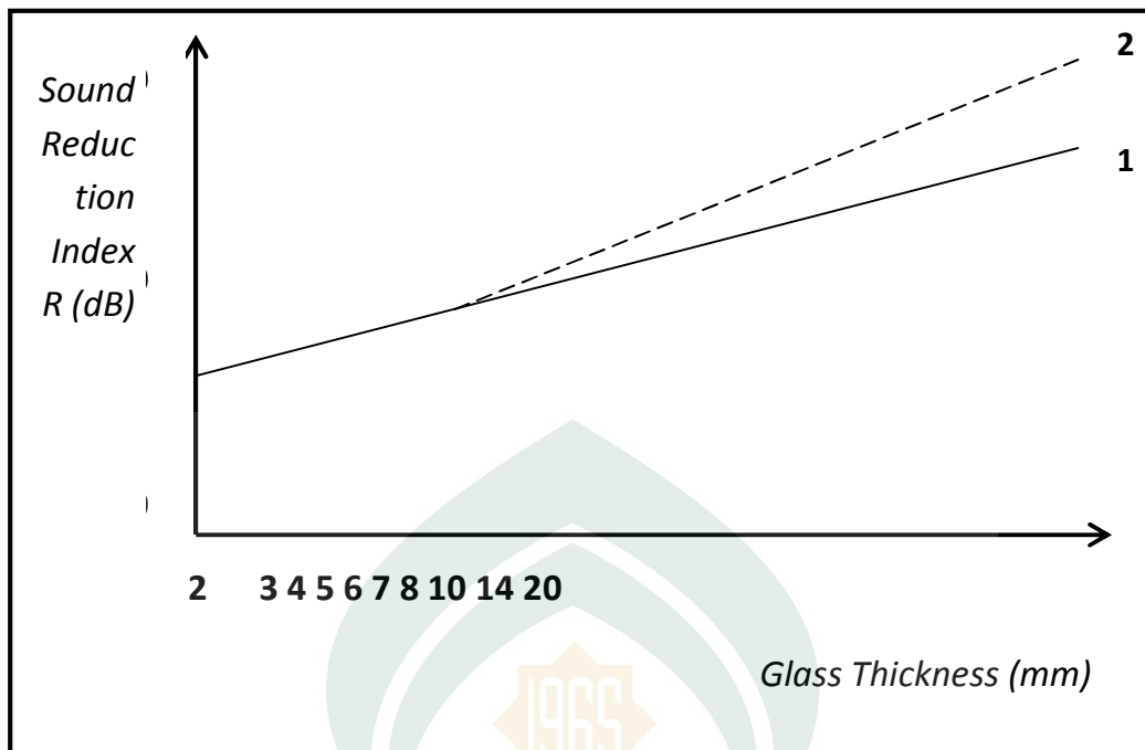
Gambar 14 : Hubungan antara ketebalan kaca dan reduksi suara Sumber : Wurm, 2007
