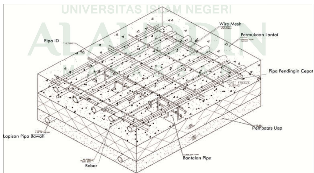
Gambar 54. Isometri Lantai Seluncur Es
