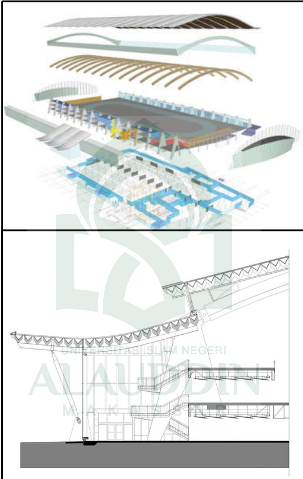
Gambar 36 :Struktur Richmond Olympic Oval Sumber :Wikipedia, diakses tanggal 11 Agustus 2016
