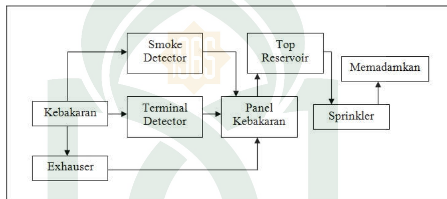
Gambar 74. Skema instalasi fire protection (Sistem bangunan pintar,2006)
