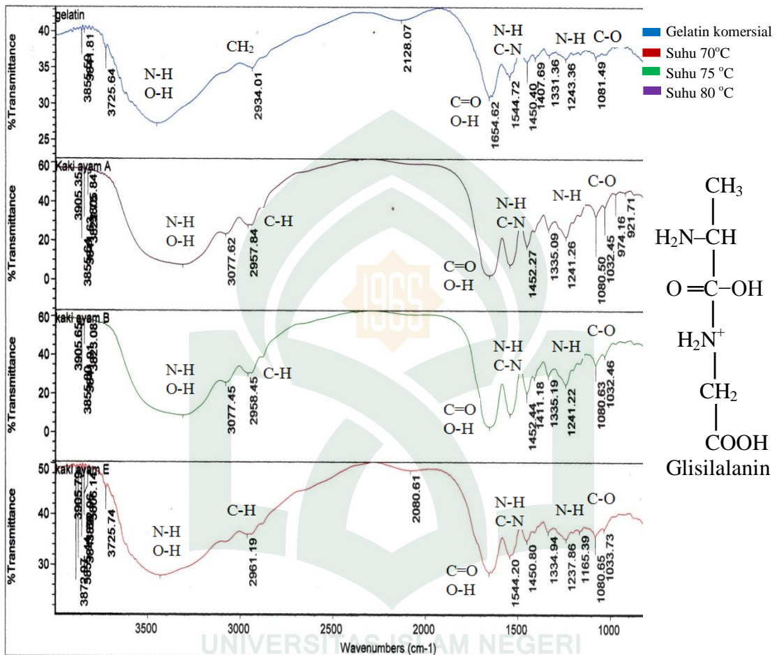
Gambar 4.7. Spektrum FTIR gelatin komersial dan tulang kaki ayam
