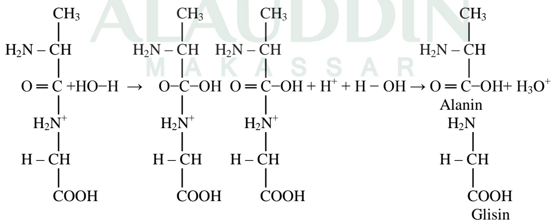
Gambar 4.2. Reaksi hidrolisis kolagen
