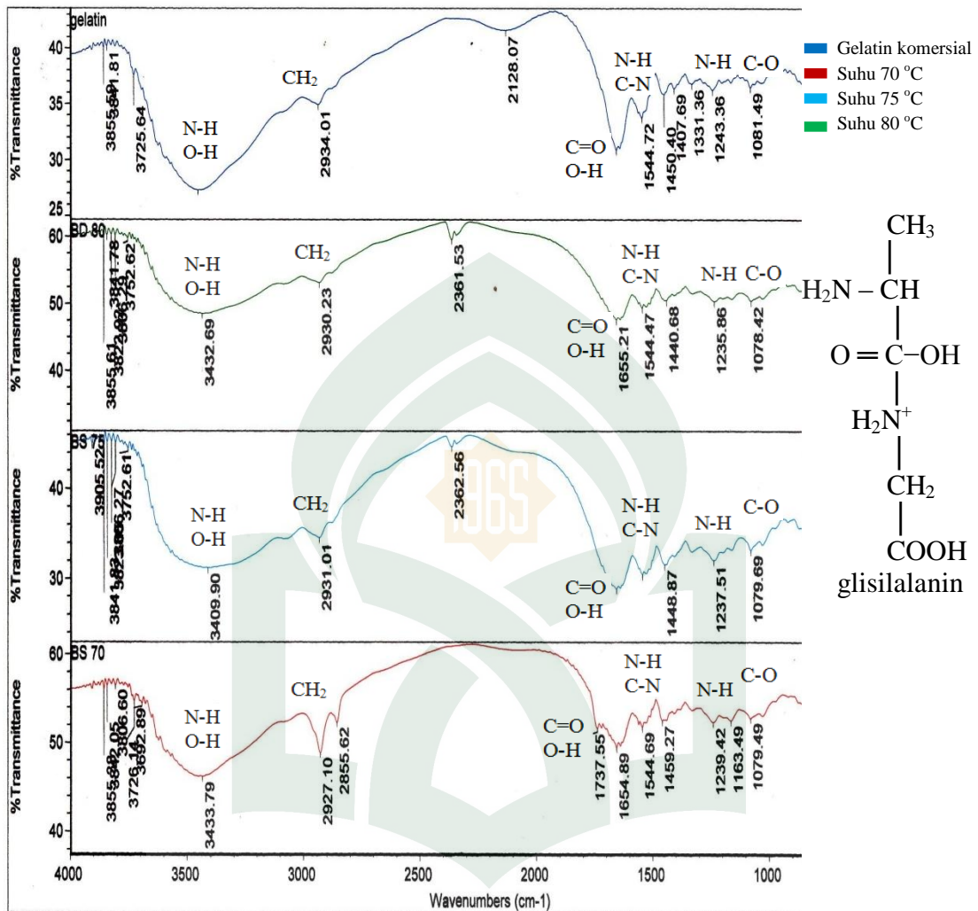
Gambar 4.8. Spektrum FTIR gelatin komersial dan kulit babi
