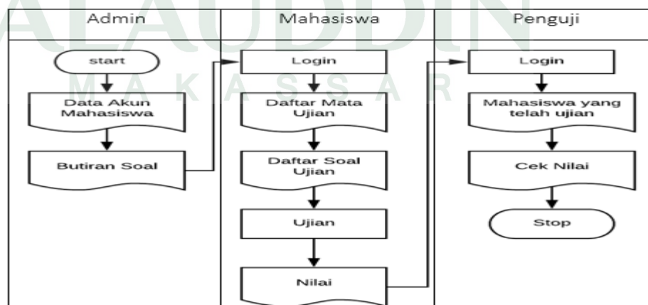
Gambar IV.2 Flowmap Diagram Sistem yang Diusulkan
