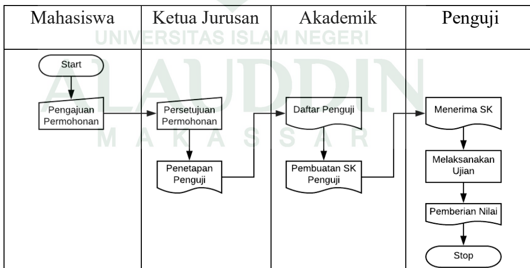
Gambar IV.1 Flowmap Diagram Sistem yang Sedang Berjalan
