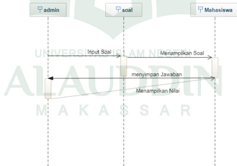
Gambar IV.6 Sequence Diagram untuk Soal
