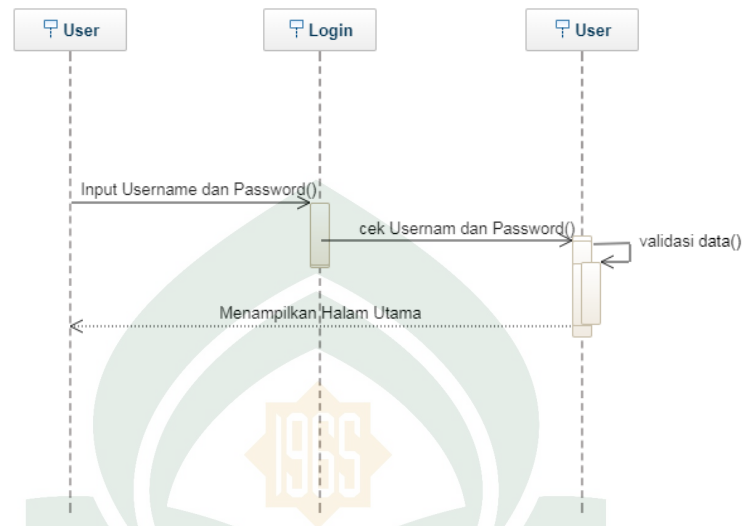
Gambar IV.5 Sequence Diagram untuk Login User
