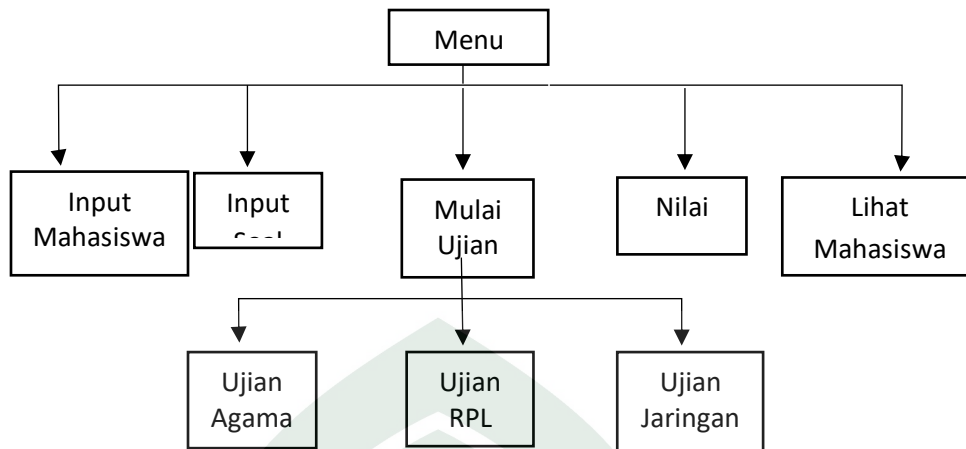
Gambar IV.10 Struktur Navigasi
