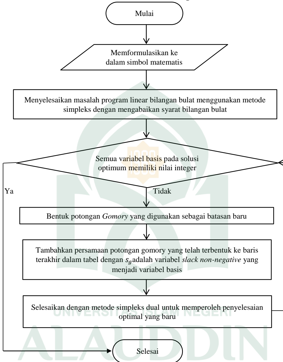
Gambar 2.1 Flowchart dari Metode Cutting Plane .
