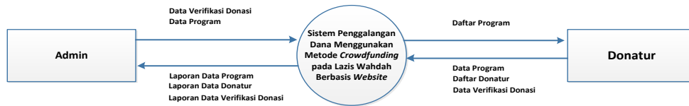
Gambar IV.3.Konteks Diagram
