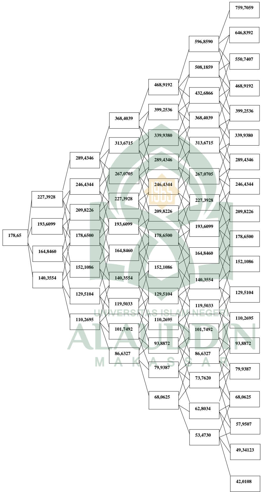
Gambar 4.2 Skema pohon multinomial harga saham 6 periode
