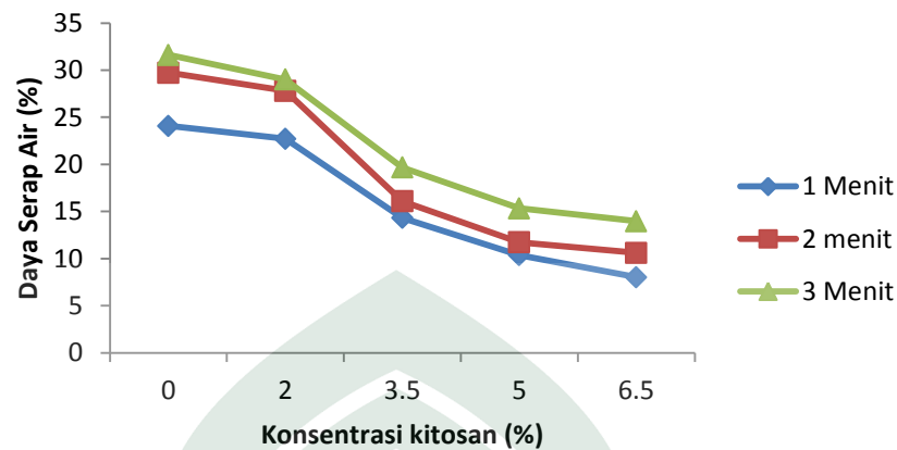
Grafik 4.1 Daya Serap Air Biofoam dari Pati Biji Nangka ( Artocarpus heterophyllus )
