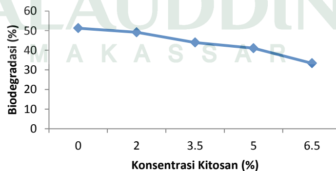
Grafik 4.2 Tingkat Biodegradasi Biofoam dari Pati Biji Nangka ( Artocarpus heterophyllus )
