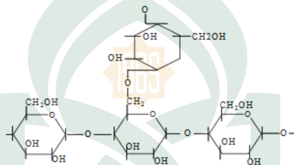
Gambar 2.2 Struktur Amilopektin
