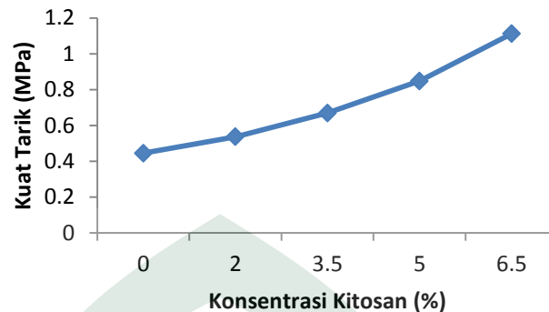
Grafik 4.3 Kuat Tarik Biofoam dari Pati Biji Nangka ( Artocarpus heterophyllus )
