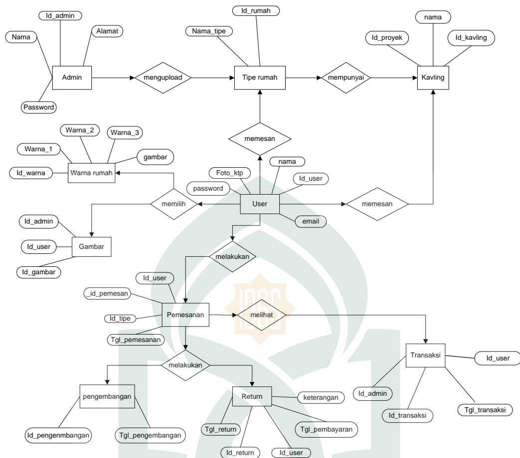
Gambar IV.10. Entity Relationship Diagram (ERD)
