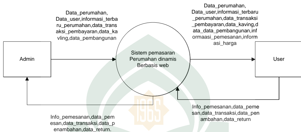
Gambar IV.4 Diagram konteks sistem pemasaran perumahan dinamis
