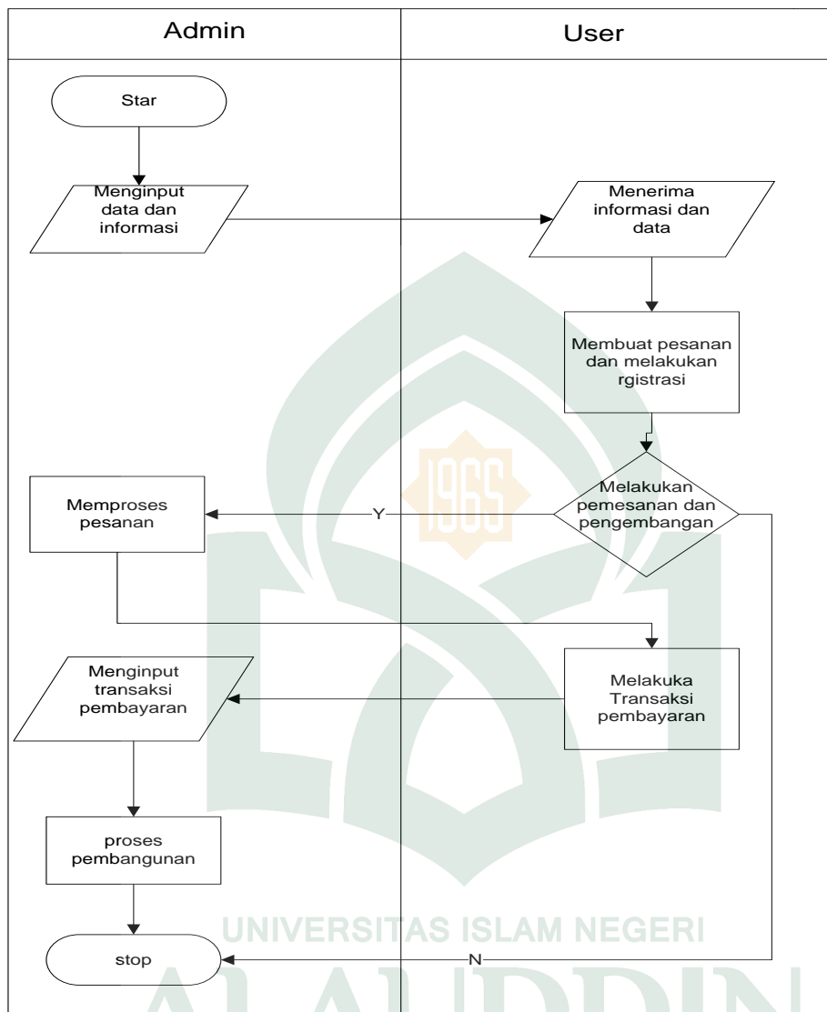
Gambar IV.3. Flowmap Diagram pada Sistem yang diusulkan.
