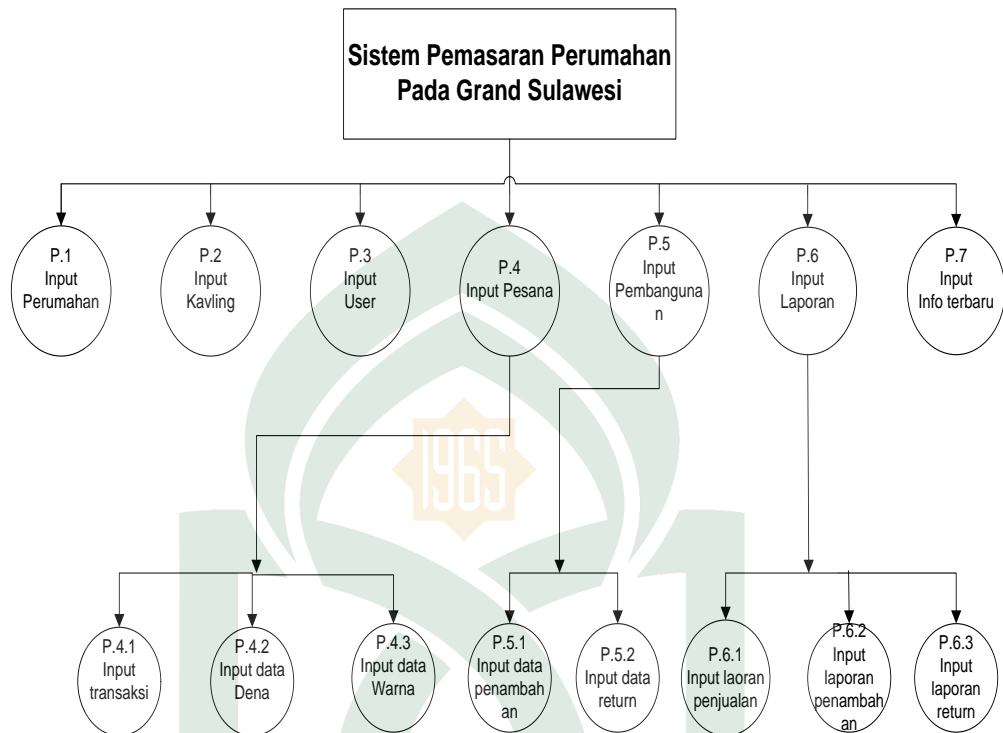
Gambar IV.5. Diagram berjenjang Sistem Pemasaran perumahan dinamis
