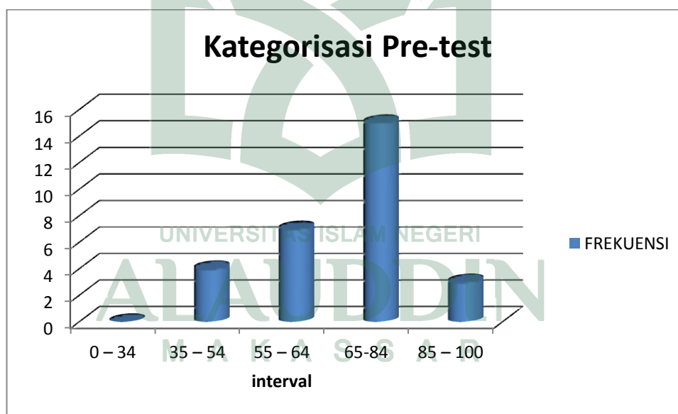
Gambar 4.1 Diagram Kategorisasi Pre-test Hasil Belajar Peserta Didik
