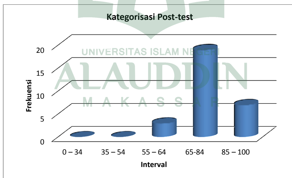
Gambar 4.2 Diagram Kategorisasi Post-test Hasil Belajar Peserta Didik
