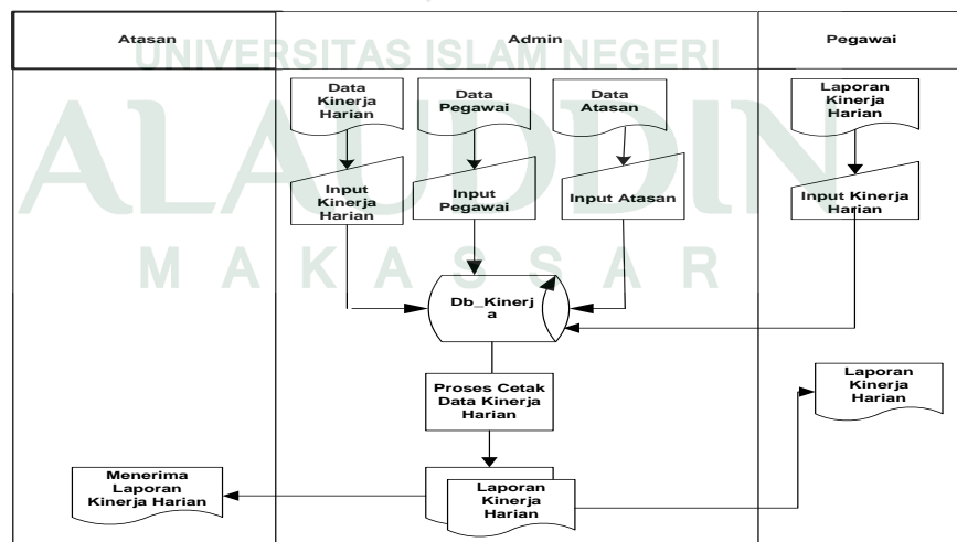
Gambar IV.2 Flowmap Sistem yang sedang Diusulkan
