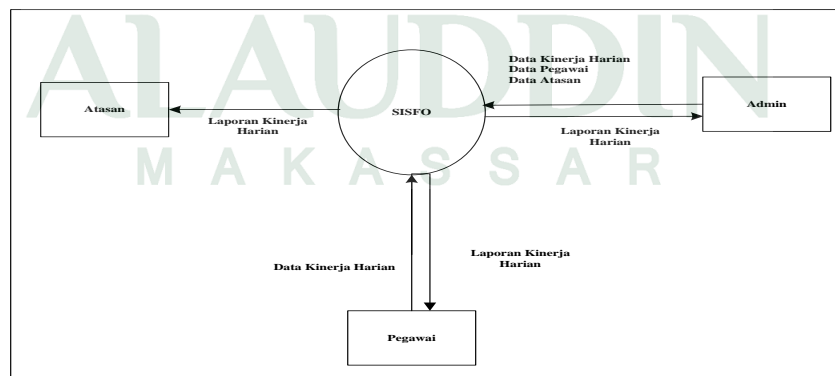
Gambar IV.3 Diagram Konteks
