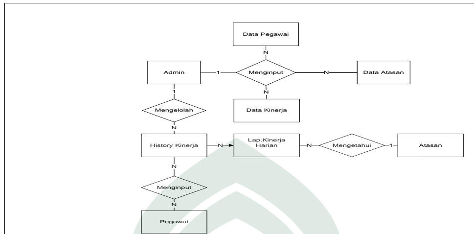
Gambar IV.7 ERD
