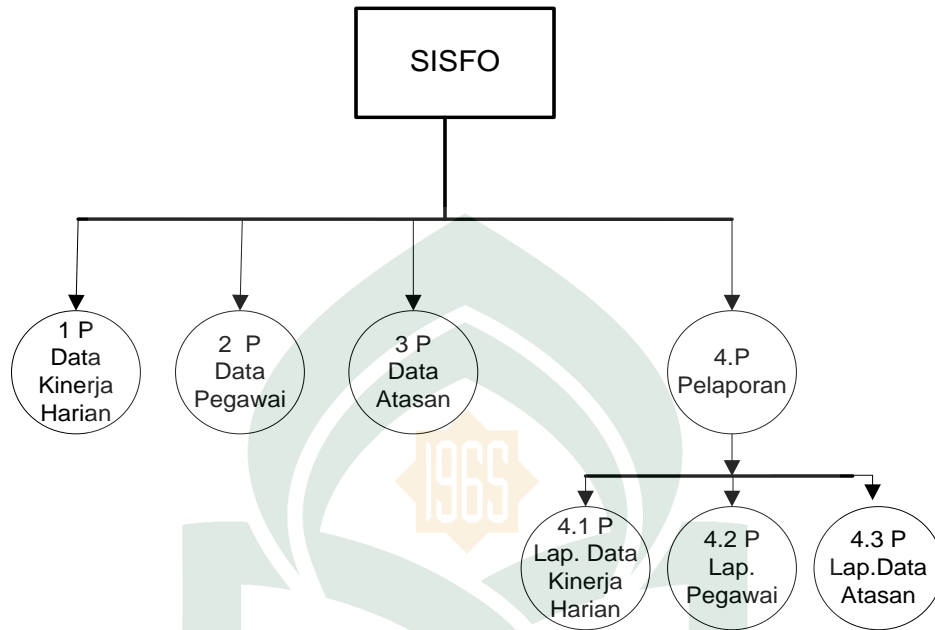
Gambar IV.4 Diagram HIPO
