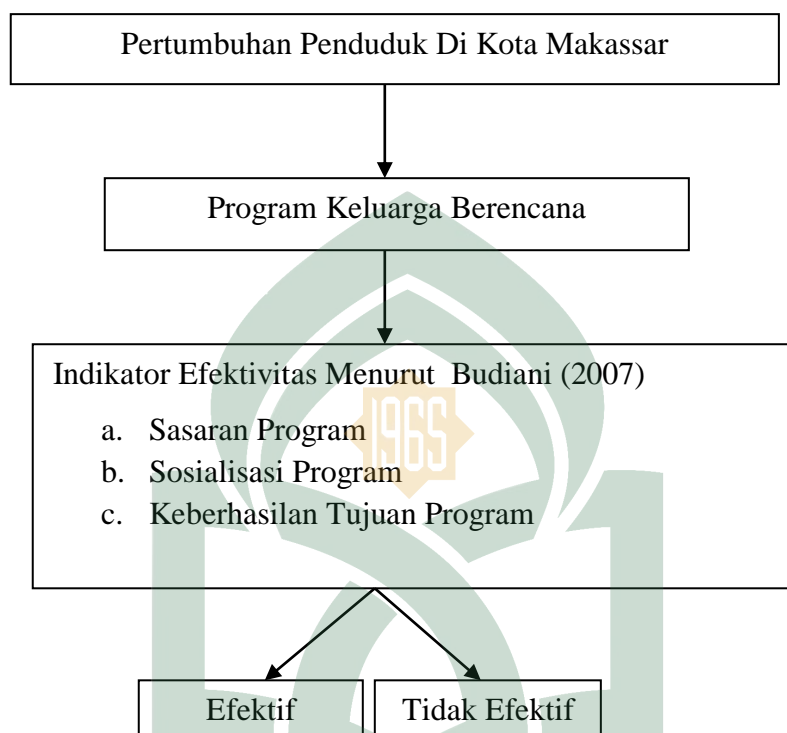
Gambar 2.1 Kerangka Pikir
