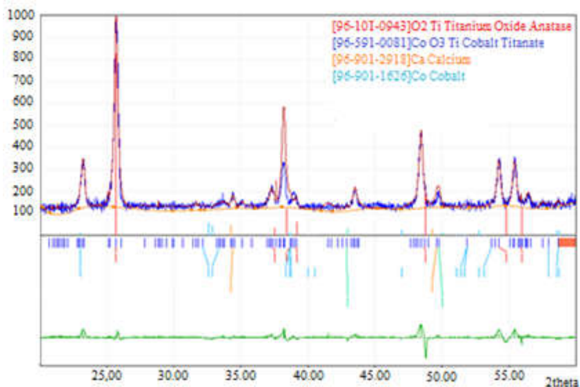
Gambar 4.1. Hubungan antara intensitas dan sudut 2\theta pada sampel Co/TiO 2
