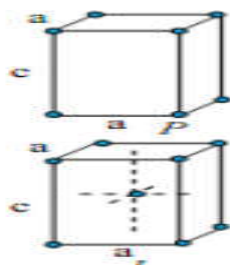
Gambar 2.7. Sistem Tetragonal
