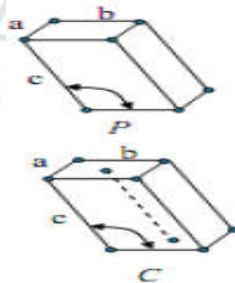
Gambar 2.9. Sistem monoklinik
