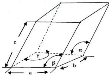
Gambar 2.10. Sistem triklinik
