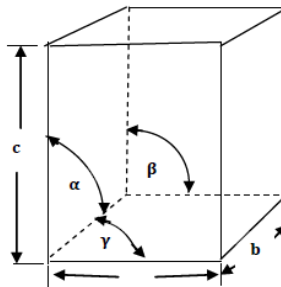
Gambar 2.11. Sistem orthorhombik
