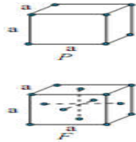
Gambar 2.6. Sistem Kubik
