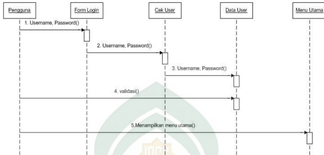
Gambar IV.6 Sequence Diagram untuk Login User
