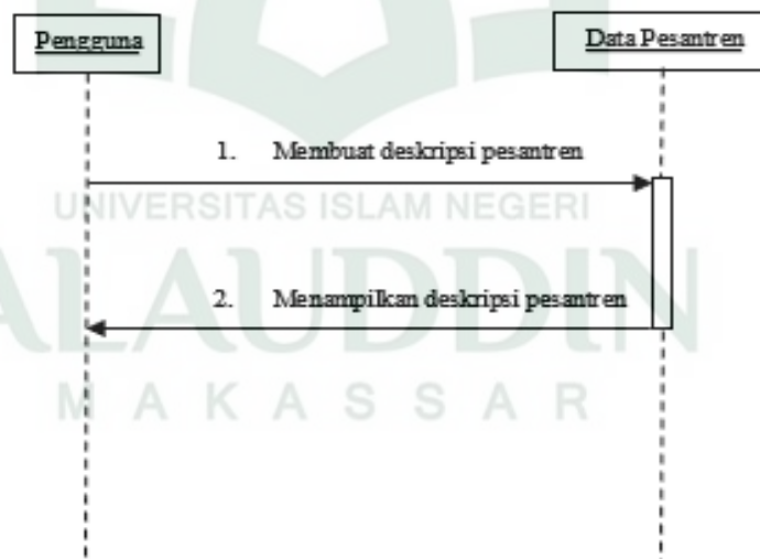
Gambar IV.7 Sequence Diagram untuk Data Pesantren dan Pengguna
