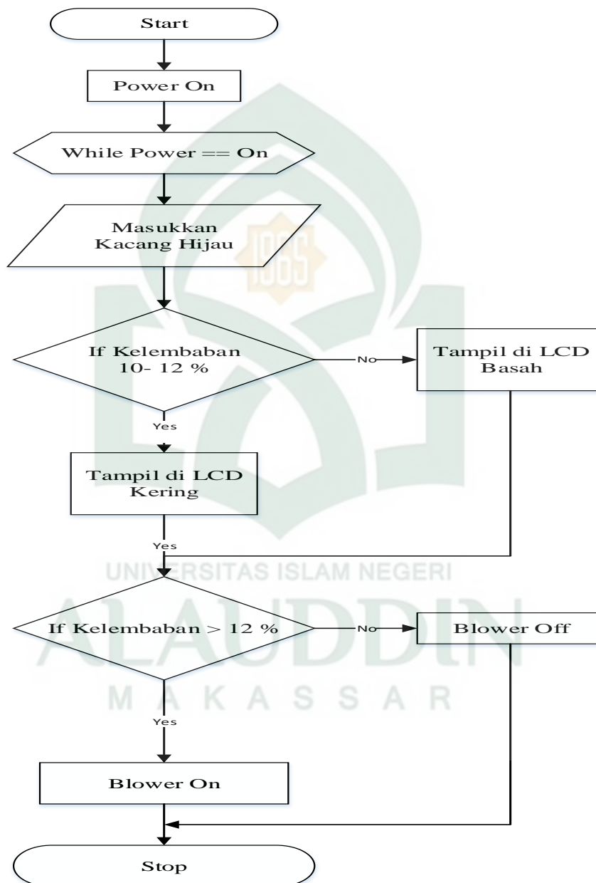
Gambar IV. 9. Flowchart Alat Pengering dan Pengupas Kacang Hijau
