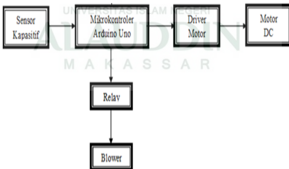
Gambar IV.1 Diagram Blok Sistem Alat
