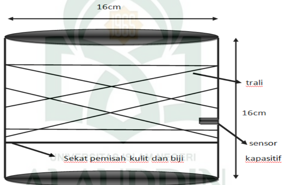
Gambar IV. 4. Rancangan Mekanik Prototype Alat Tampak Dalam
