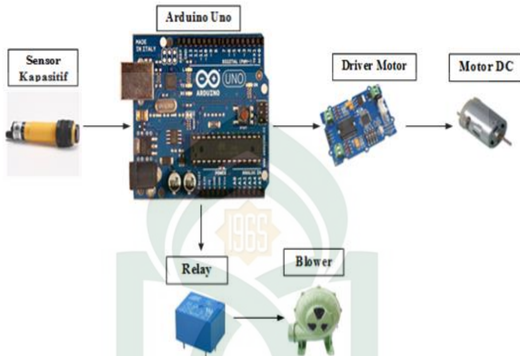
Gambar IV.2 Susunan Alat yang digunakan
