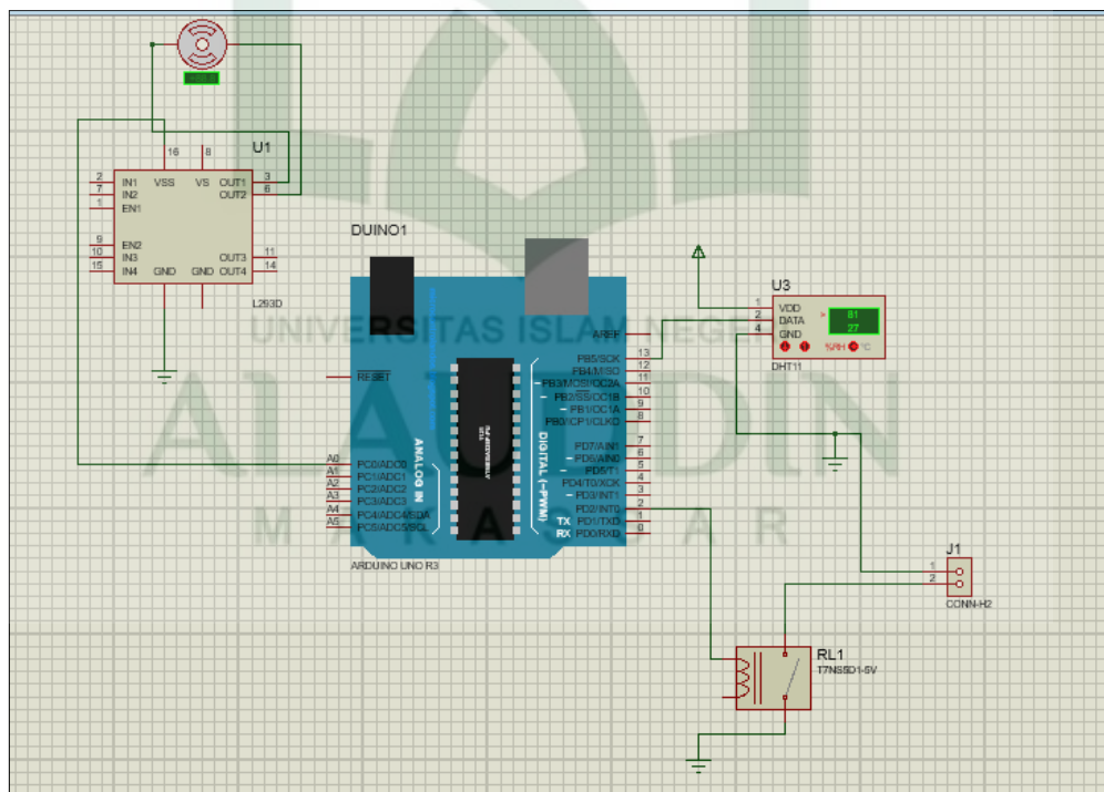
Gambar IV.5. Rancangan Sistem Rangkaian Elektronika
