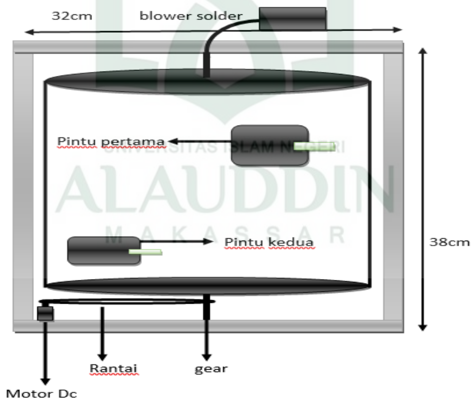
Gambar IV. 3. Rancangan Mekanik Prototype Alat Tampak Luar
