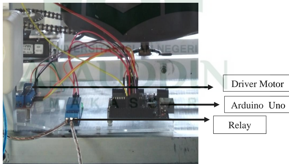
Gambar V.2. Rangkaian Sistem Elektronika
