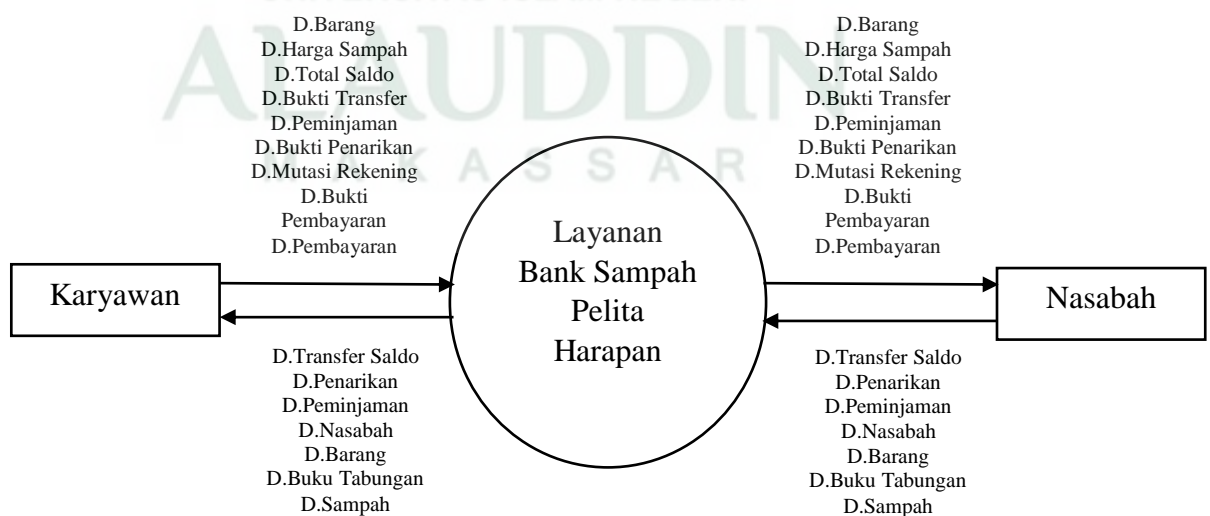
Gambar IV.3 Diagram Konteks Layanan Bank Sampah Pelita Harapan
