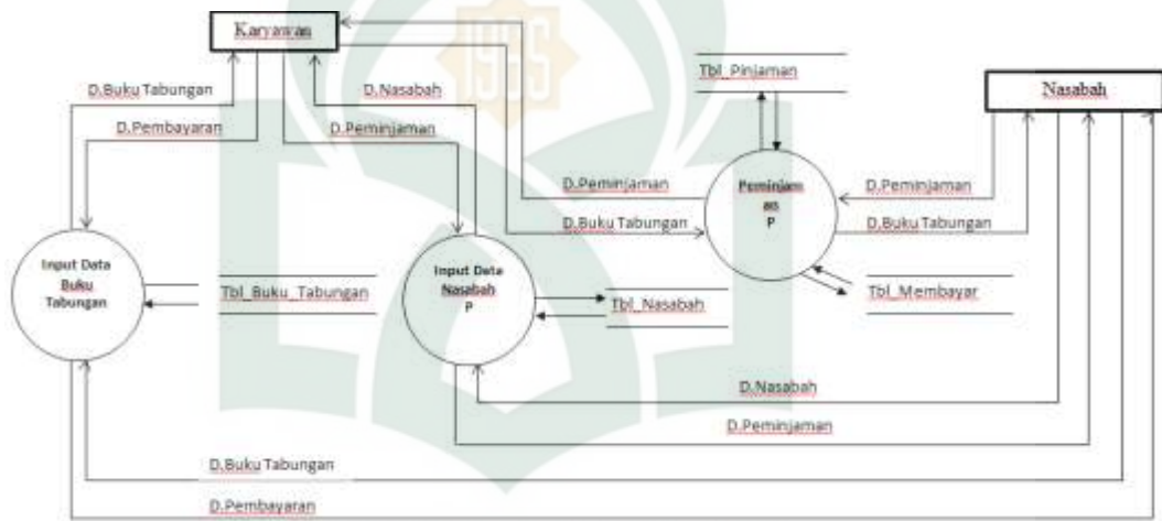
Gambar IV.11 Data Flow Diagram (DFD) Level 2 Layanan Peminjaman
