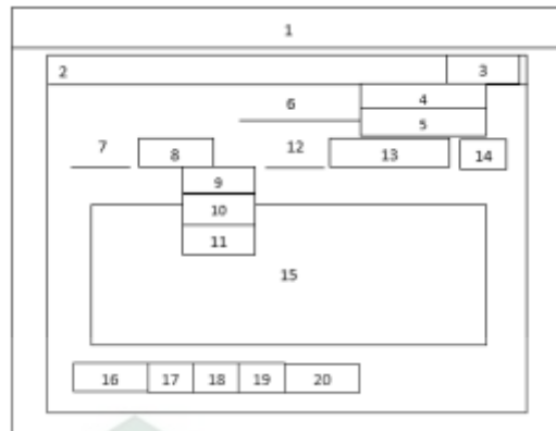
Gambar IV.17 Perancangan Aplikasi Pencarian Nasabah
