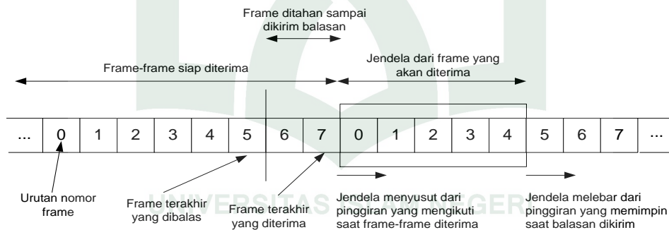
Gambar II.4 Jendela Penggeseran Menurut Perspektif Penerima (Stallings, 2001a)
