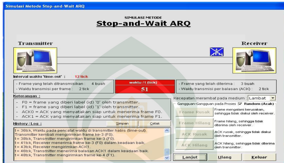
Gambar V.9 Tampilan frame rusak pada Stop and Wait ARQ
