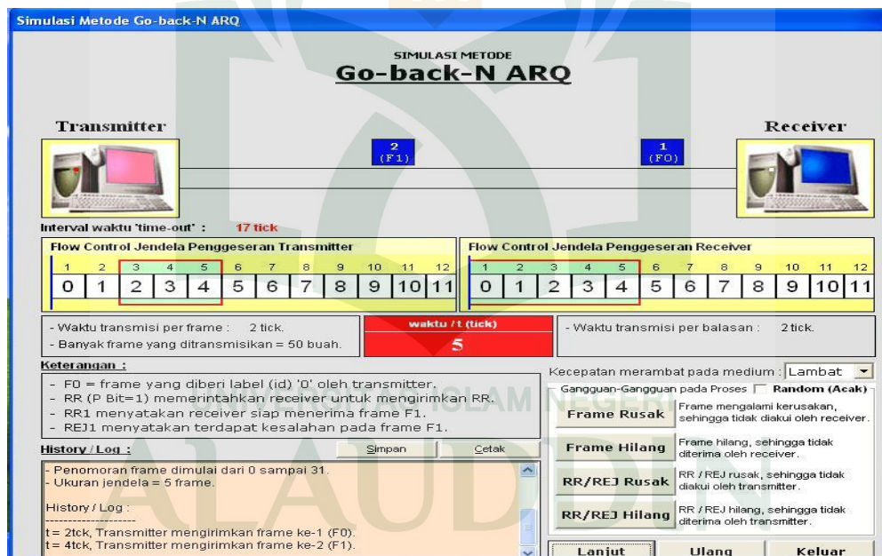
Gambar V.5 Tampilan Jendela Simulasi Go Back N ARQ
