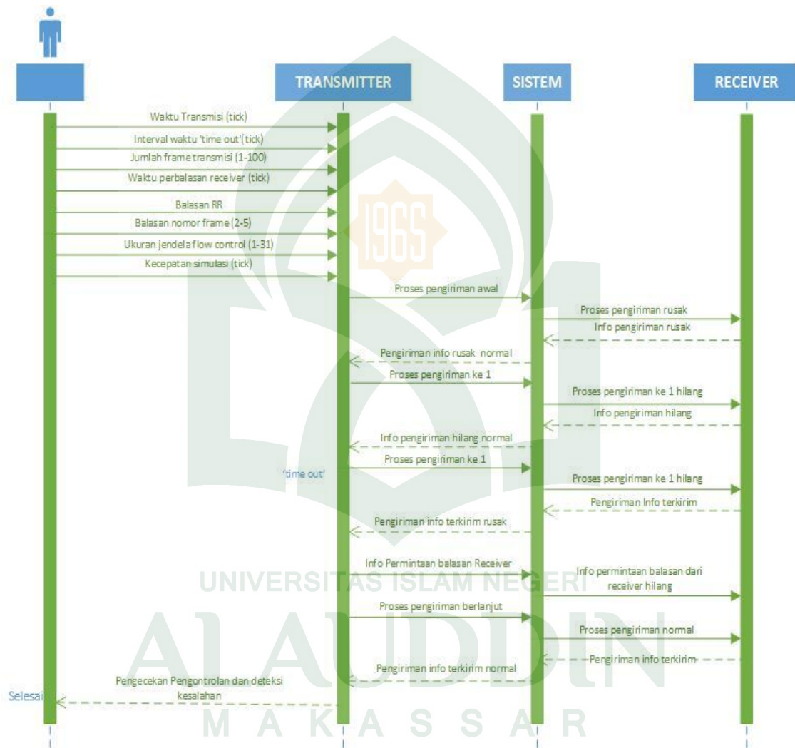
Gambar IV.9 Sequence Diagram Metode Go-Back- N ARQ Tidak Normal
