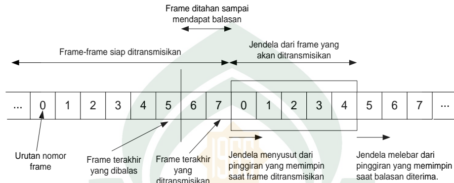
Gambar II.3 Jendela Penggeseran Menurut Perspektif Pengirim (Stallings, 2001a)
