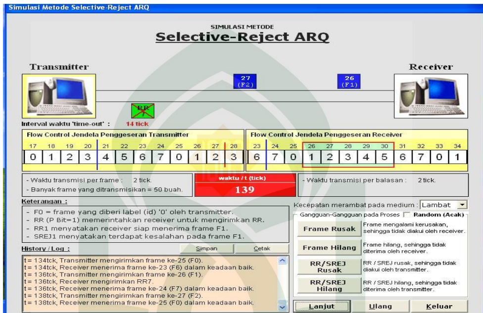
Gambar V.14 Tampilan RR/SREJ Rusak pada Selective Reject ARQ
