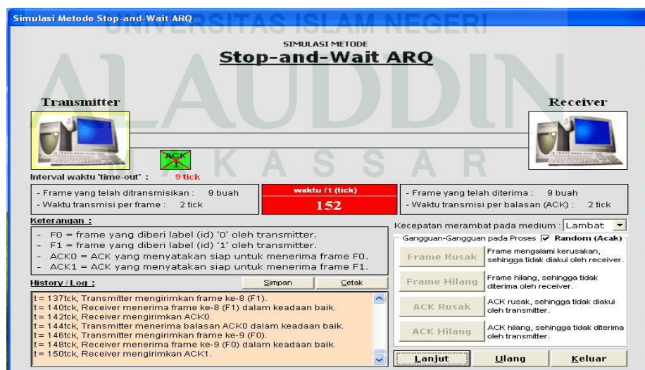
Gambar V.10 Tampilan ACK rusak pada Stop and Wait ARQ
