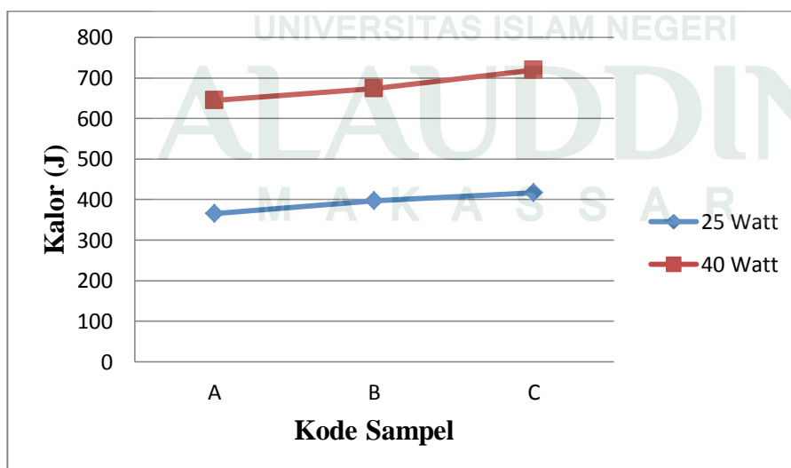
Grafik IV.3 Grafik uji perpindahan kalor
