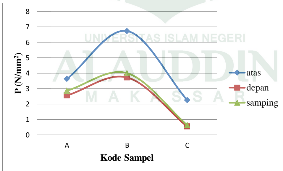
Grafik IV.2 Grafik pengujian kuat tekan
