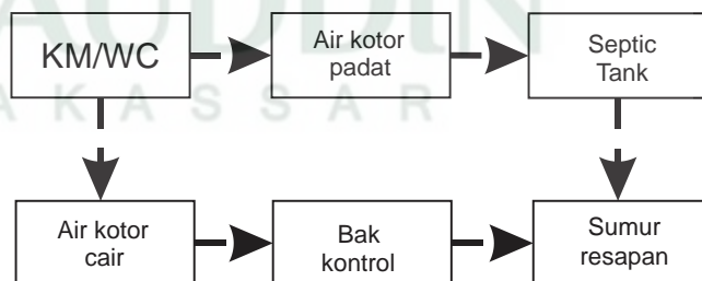
Skema IV. 1 Alur pembuangan Air kotor KM/WC Sumber : Hartono, Acuan perancangan, 2012
