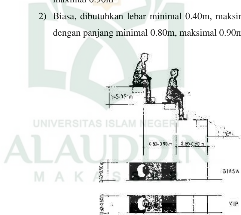
Gambar IV. 15 Standar tempat duduk pada tribun Sumber: Tata cara perencanaan teknik bangunan gedung olahraga, Mei 2015
