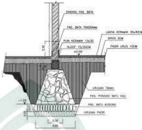
Gambar IV. 28 Pondasi batu kali Site.com, diakses 5 mei 2015
