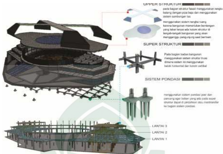
Gambar V. 8 Konsep Struktur (Olah Desain : 2015)
