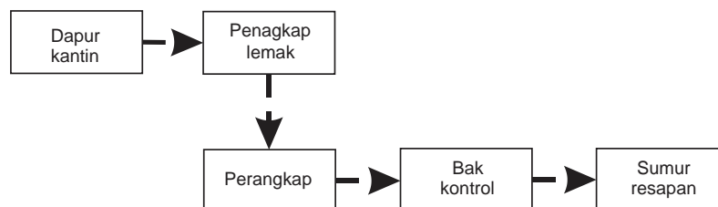
Skema IV. 2 Alur pembuangan air kotor dapur kantin Sumber : Hartono, Acuan perancangan, 2012
