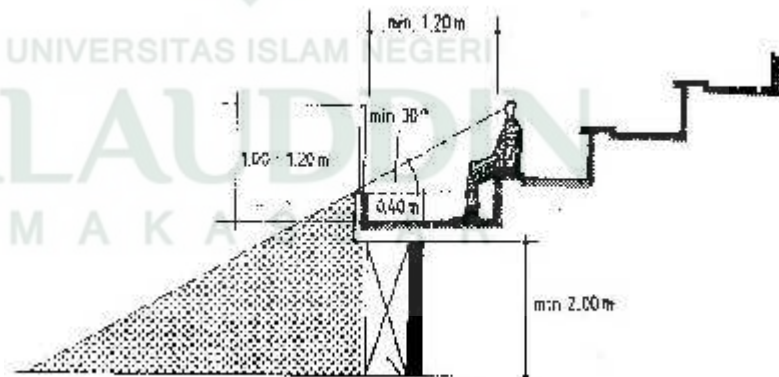
Gambar IV. 14 Pemisah antara tribun dan arena
