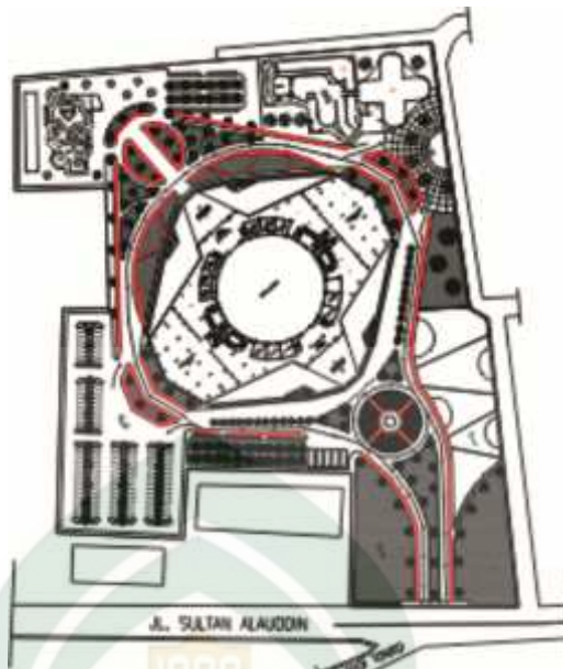
Gambar VI. 3 Sirkulasi Pejalan kaki Pada Tapak (Olah Desain : 2015)
