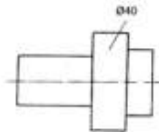
Gambar 91 Ukuran diameter dengan garis petunjuk
