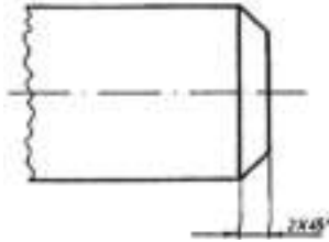
Gambar 66 Kemiringan
