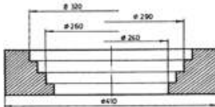
Gambar 55 Garis ukur sebagian
