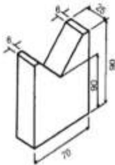
Gambar 13 VEE Blok
