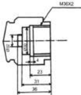
Gambar 75 Ukuran-ukuran terhadap bidang referensi
