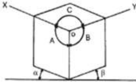
Gambar 12 Proyeksi dimetri
