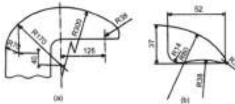
Gambar 86 Memberi ukuran dengan jari-jari
