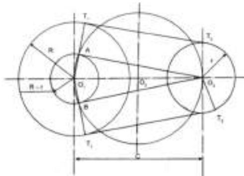
Gambar 21 Sabuk terbuka
