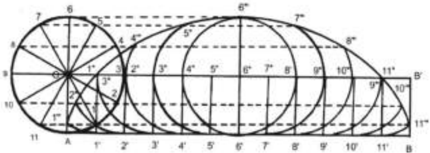
Gambar 32 Lengkung cycloida
