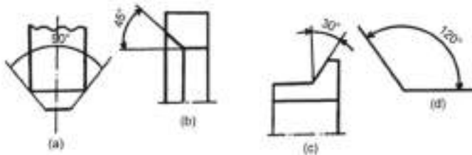
Gambar 92 Pemberian ukuran sudut
