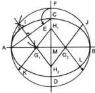
Gambar 28 Bulat lonjong
