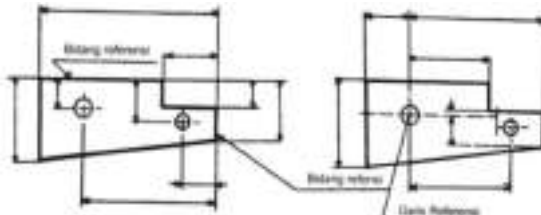
Gambar 77 Ukuran-ukuran terhadap bidang atau garis referensi yang ditunjuk
