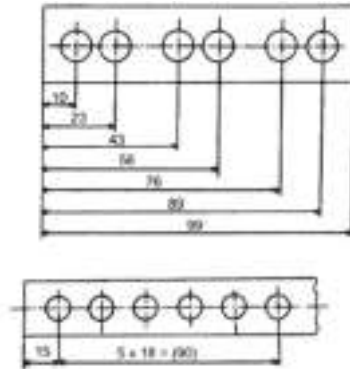
Gambar 78 Memberi ukuran bagian-bagian Yang berjarak sama
