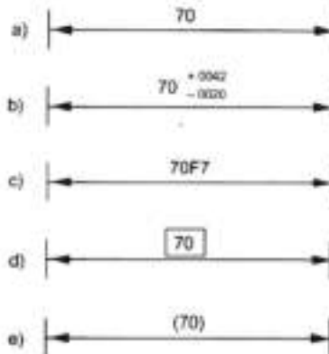
Gambar 41 Macam-macam jenis ukuran dan toleransi
