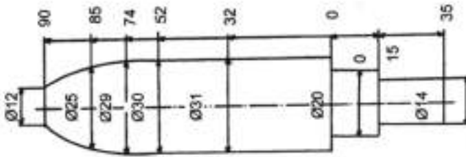
Gambar 102 Ukuran-ukuran yang berurutan
