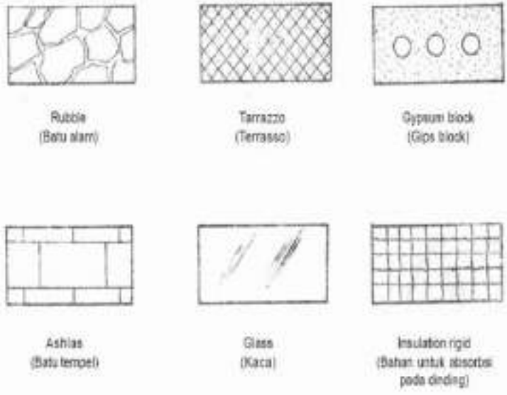
Gambar 106 Jenis Arsiran
