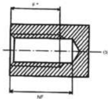
Gambar 44 Dimensi fungsional dan dimensi Tidak fungsional
