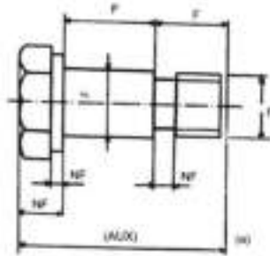
Gambar 43 Dimensi fungsional dan dimensi Tidak fungsional
