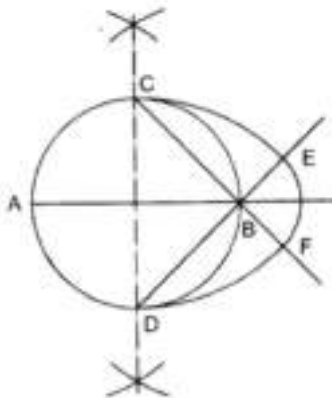
Gambar 25 Menggambar bulat telur jika lebaranya ditentukan (Cara I)
