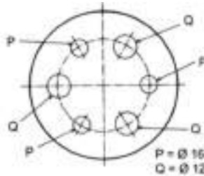
Gambar 70 Memberi ukuran dengan huruf-huruf referensi
