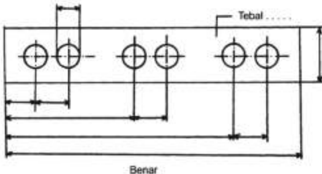
Gambar 103 Ukuran kombinasi/gabungan
