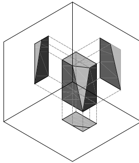
Gambar 1 Proyeksi Eropa
