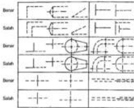
Gambar 4 Gambar garis gores dan garis bertitik
