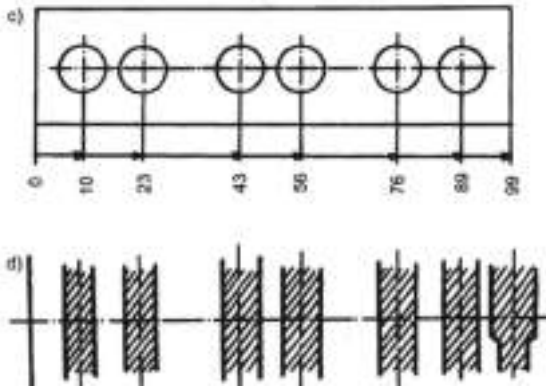
Gambar 101 c dan d ukuran-ukuran dan diagram toleransinya
