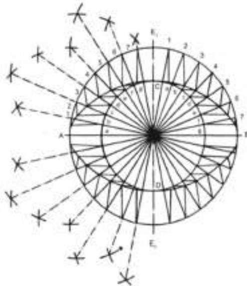
Gambar 29 Menggambar elips (Cara I)
