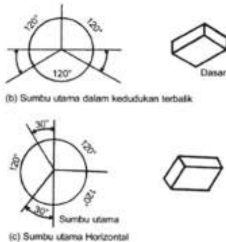
Gambar 5 Kedudukan sumbu-sumbu isometri
