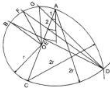
Gambar 12 Membagi tiga sudut sembarang
