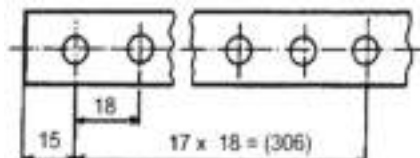
Gambar 79 Memberi ukuran bagian-bagian Yang berjarak sama
