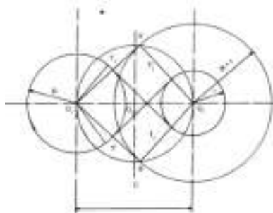
Gambar 22 Sabuk menyilang
