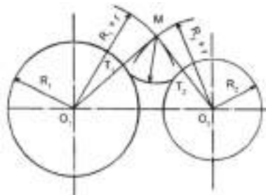
Gambar 23 Sebuah busur meyinggung Dua buah lingkaran
