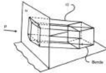
Gambar 19 Proyeksi miring
