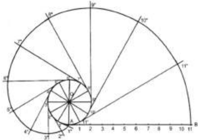
Gambar 31 Lengkung evolvent
