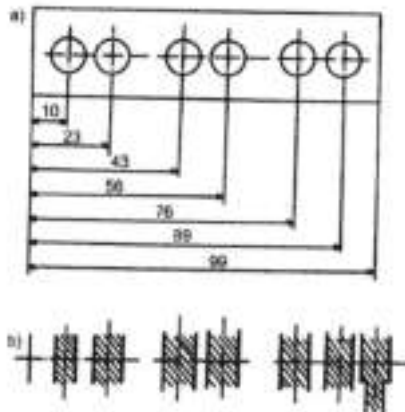
Gambar 100 a dan b ukuran dan diagram toleransinya
