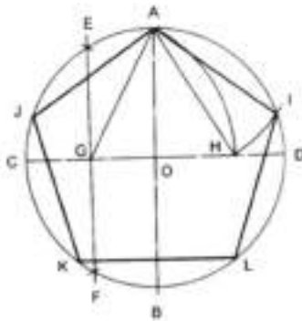
Gambar 14 Segilima teratur dalam sebuah lingkaran tertentu
