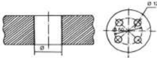
Gambar 81 Memberi ukuran lubang
