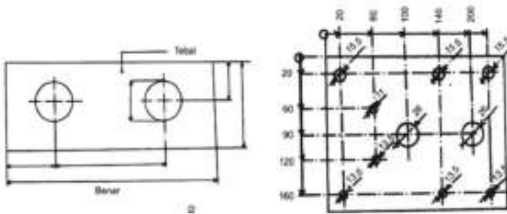
Gambar 104 Memberi ukuran dengan koordinat-koordinat
