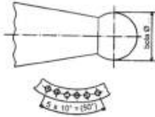
Gambar 80 Memberi ukuran bagian-bagian Yang berjarak sama
