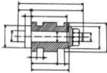
Gambar 97 Memberi ukuran bagian-bagian yang disusun
