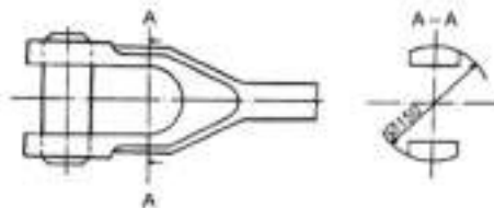
Gambar 89 Diameter diperlukan untuk proses permesinan
