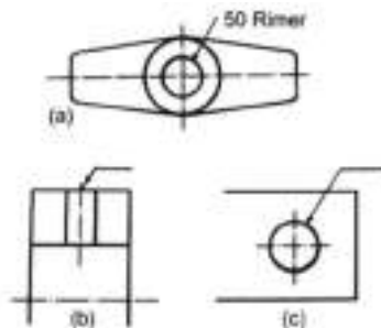
Gambar 50 Memberi ukuran lubang
