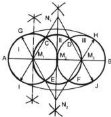
Gambar 27 Gambar bulat lonjong
