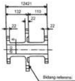
Gambar 76 Ukuran-ukuran terhadap bidang referensi yang ditunjuk
