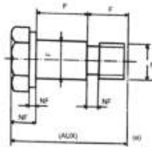
Gambar 45 Dimensi fungsional dan dimensi Tidak fungsional
