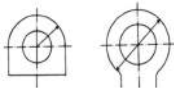
Gambar 88 Memberi ukuran dengan jari-jari dan diameter
