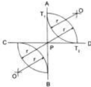
Gambar 19 Sebuah busur yang meyinggung Dua garis tegak lurus
