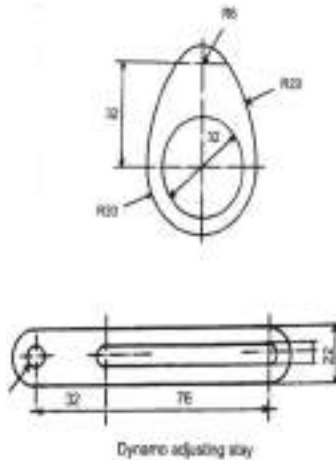
Gambar 21 Menggambar nok dan Dynamo adjusting stay
