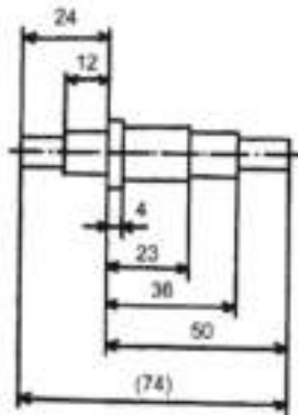
Gambar 74 Ukuran-ukuran terhadap bidang referensi
