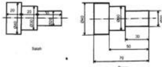
Gambar 96 Memberi ukuran bagian-bagian berbentuk silinder
