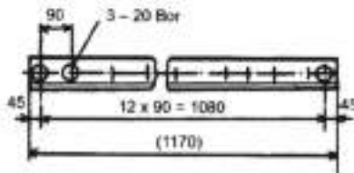
Gambar 93 Ukuran-ukuran bagian-bagian yang sama
