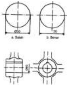
Gambar 95 Diameter dalam dengan alur pasak
