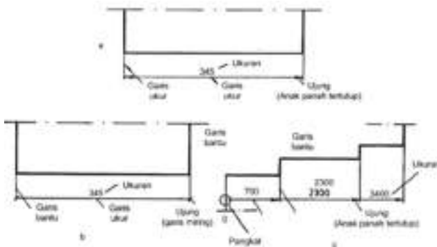
Gambar 40 Ujung dan pangkal garis ukur
