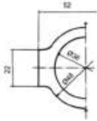
Gambar 90 Diameter pada separuh dari bagian simetris
