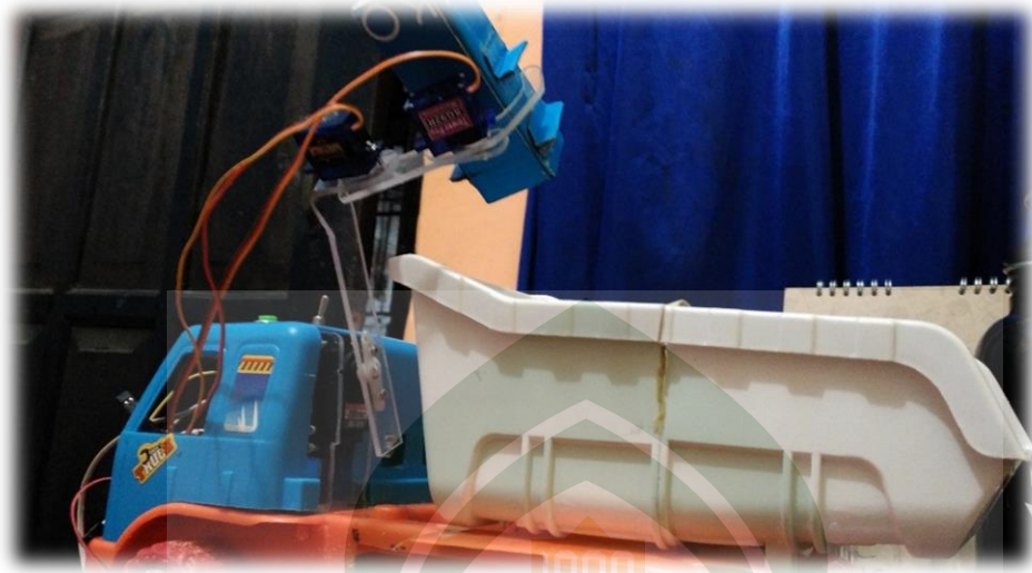
Gambar V.3 Pengujian Servo Sendi Lengan Utama.
