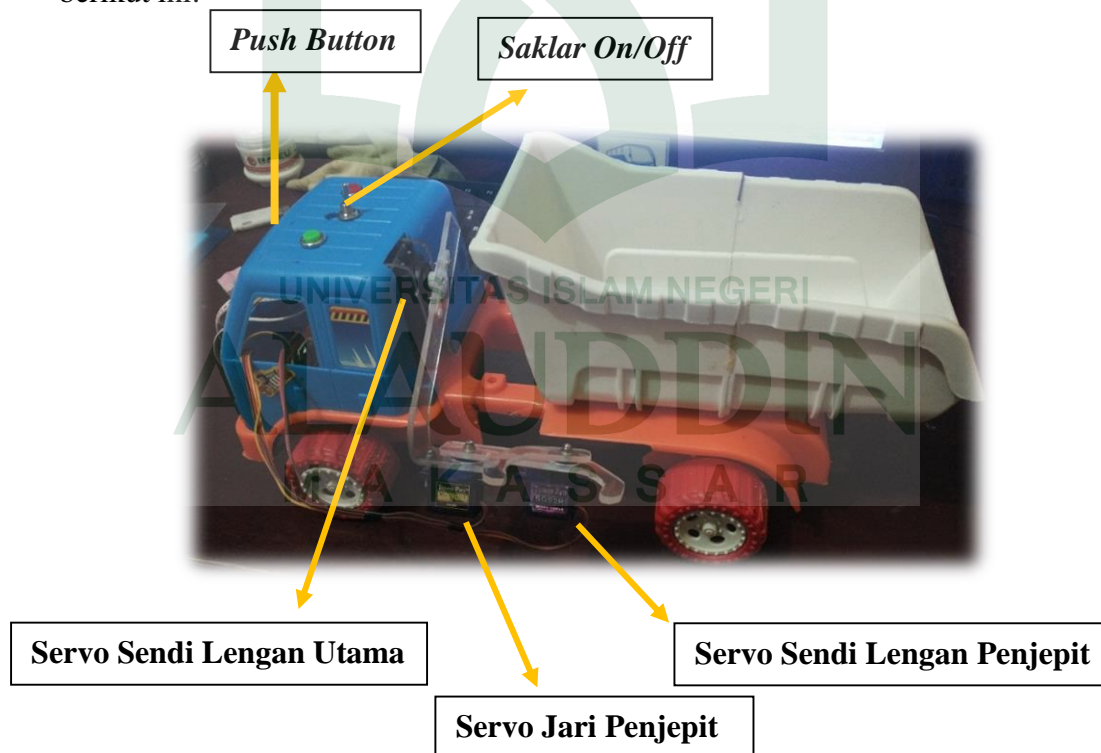
Gambar V.1 Hasil Rancangan Lengan Robot.
