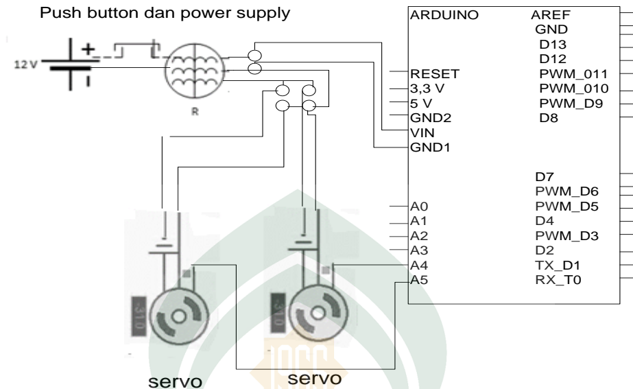
Gambar IV.3 Rancangan Desain Alat.
