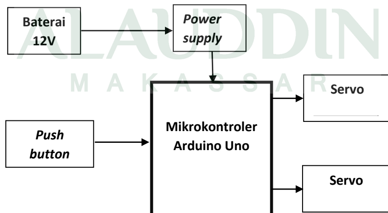
Gambar IV.1 Diagram Blok Sistem Alat.
