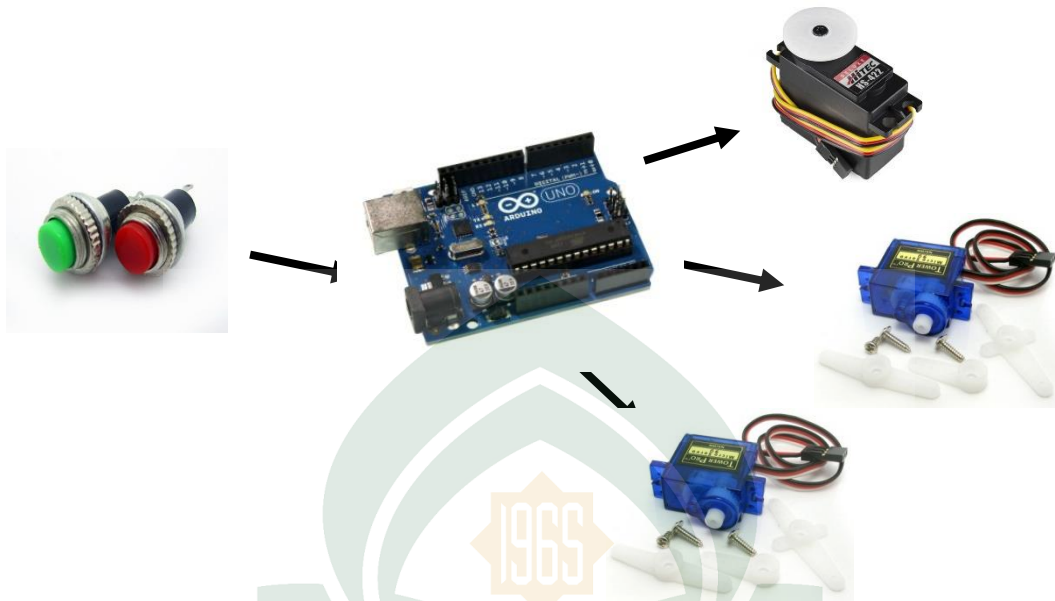
Gambar IV.2 Susunan Alat yang Digunakan.
