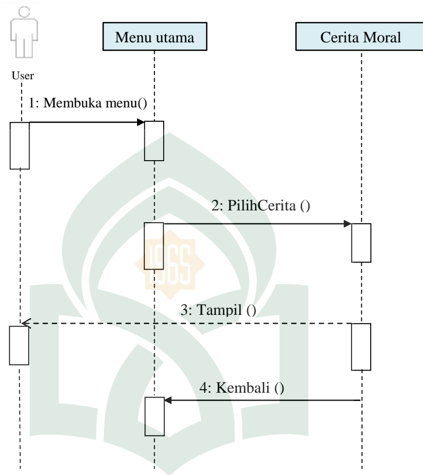
Gambar IV. 7 Sequence Diagram untuk Menu Cerita Moral
