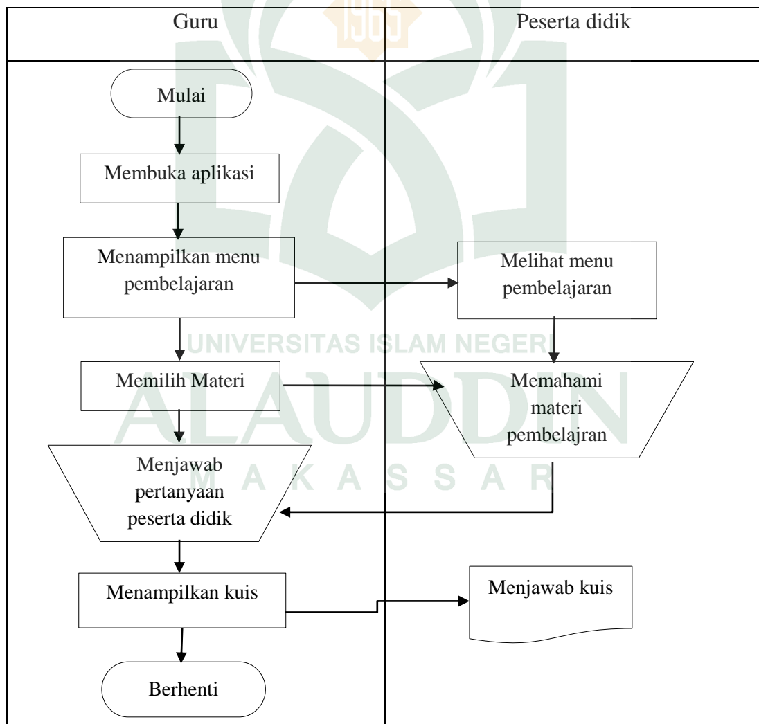
Gambar IV.2 Flowmap Diagram Sistem yang Sedang diusulkan
