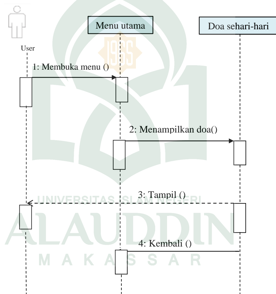
Gambar IV. 5 Sequence Diagram untuk Menu doa sehari- hari
