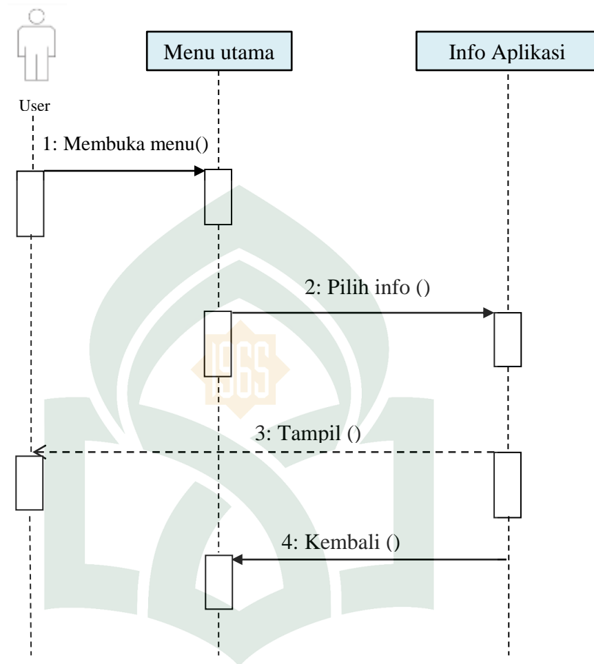
Gambar IV. 9 Sequence Diagram untuk Menu Info Aplikasi
