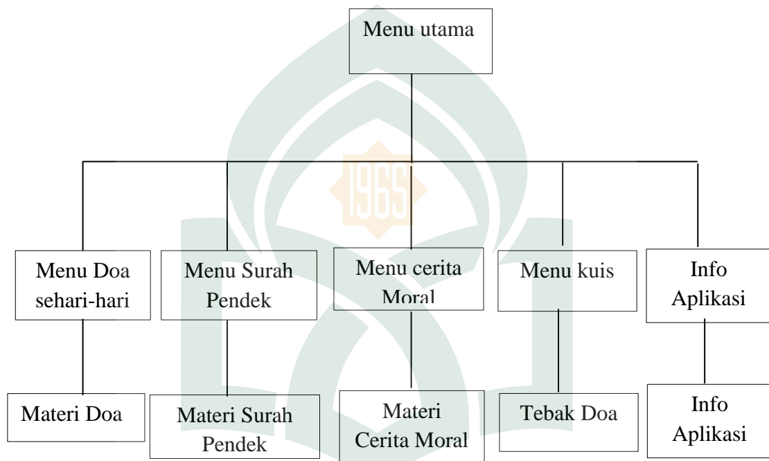
Gambar IV. 10 Struktur Navigasi
