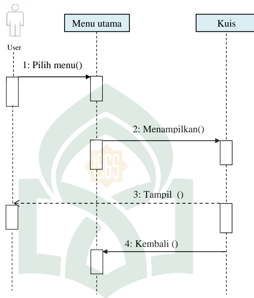
Gambar IV. 8 Sequence Diagram untuk Menu Kuis
