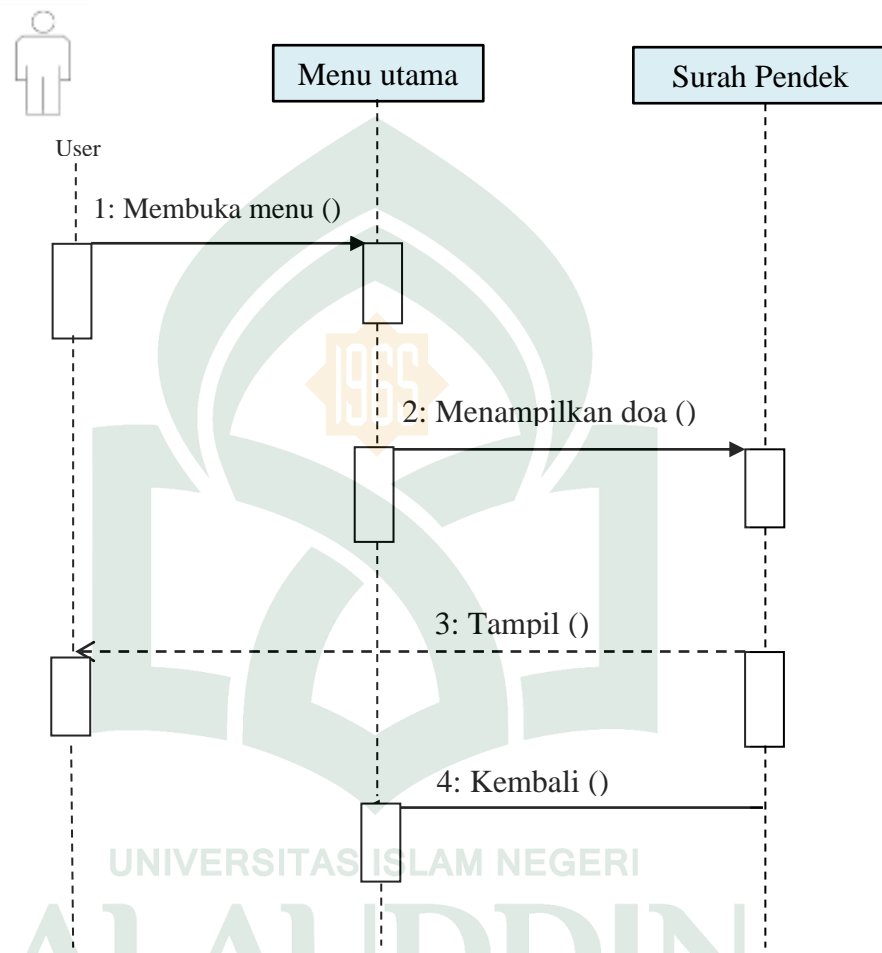
Gambar IV. 6 Sequence Diagram untuk Menu Surah Pendek
