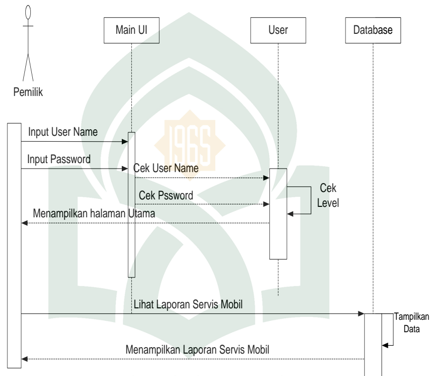
Gambar IV. 7 Sequence Diagram Pemilik
