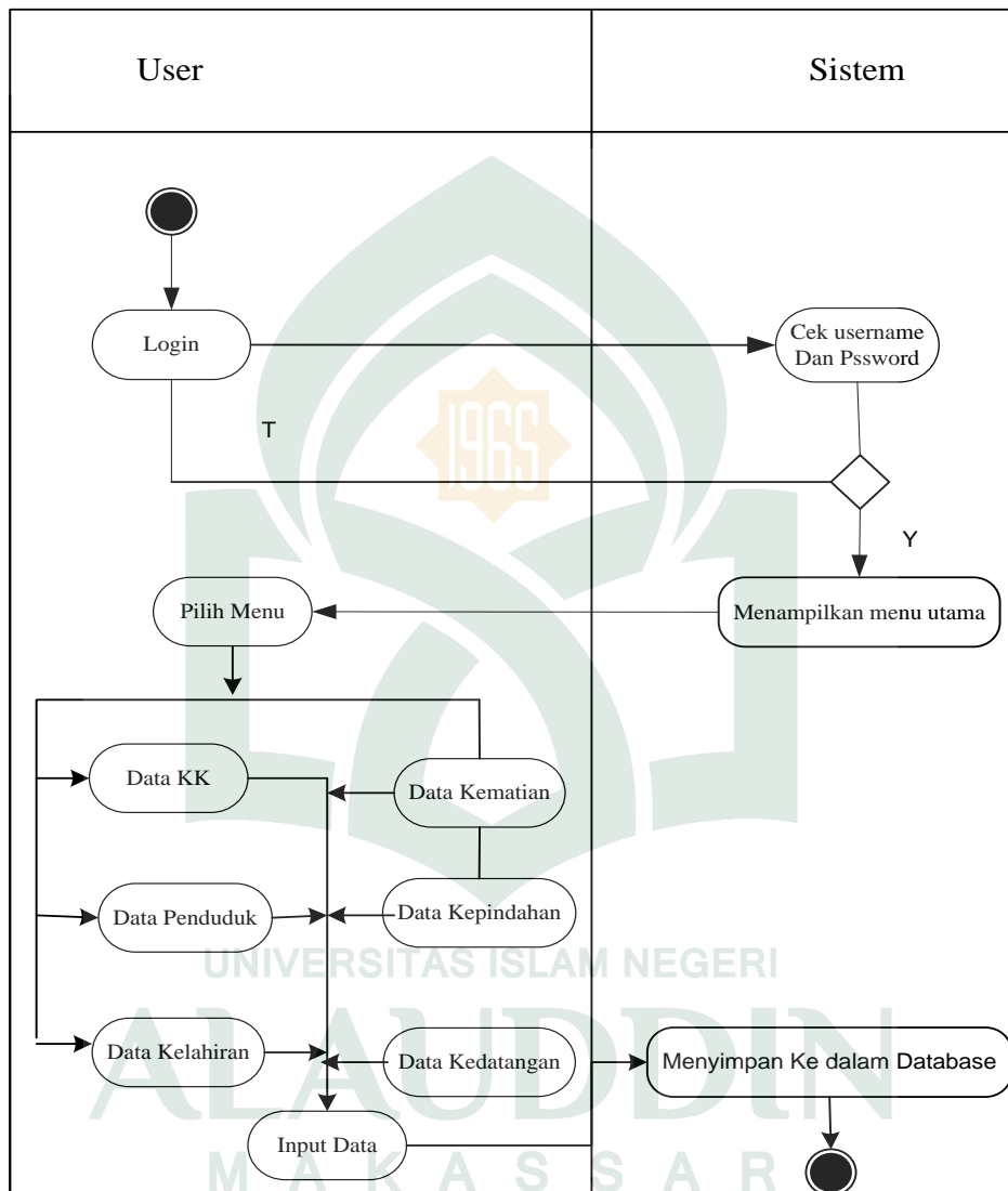
Gambar IV. 4 Activity diagram BPS Kabupaten
