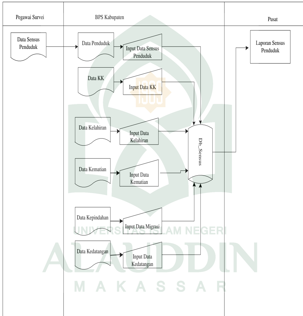
Gambar IV. 2 Flowmap Sistem yang sedang Diusulkan
