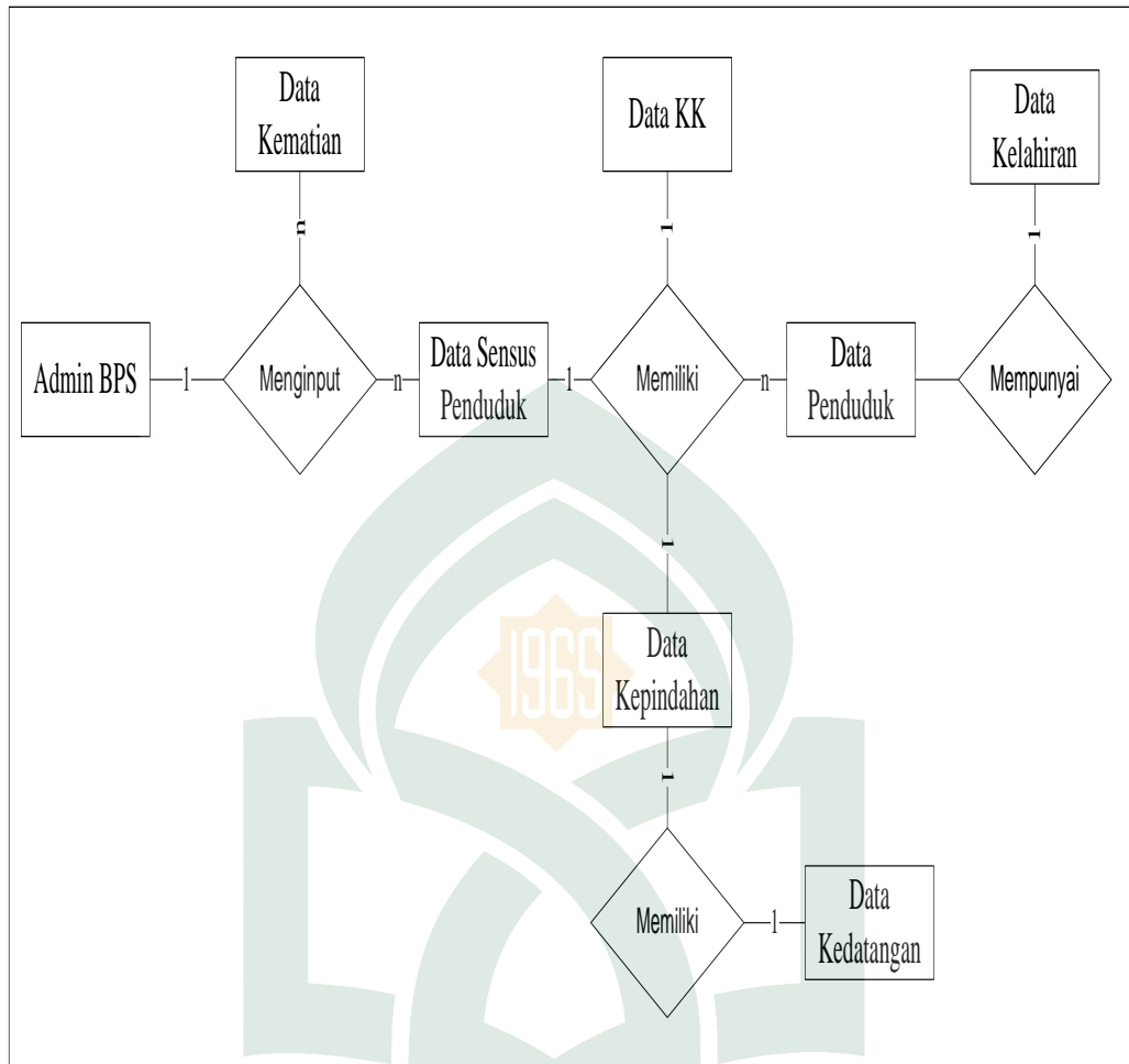
Gambar IV. 8 ERD
