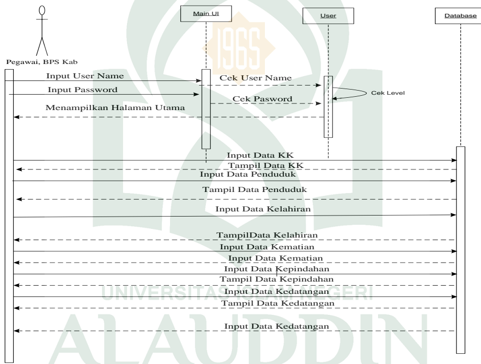
Gambar IV. 6 Sequence Diagram Admin dan BPS Kabupaten
