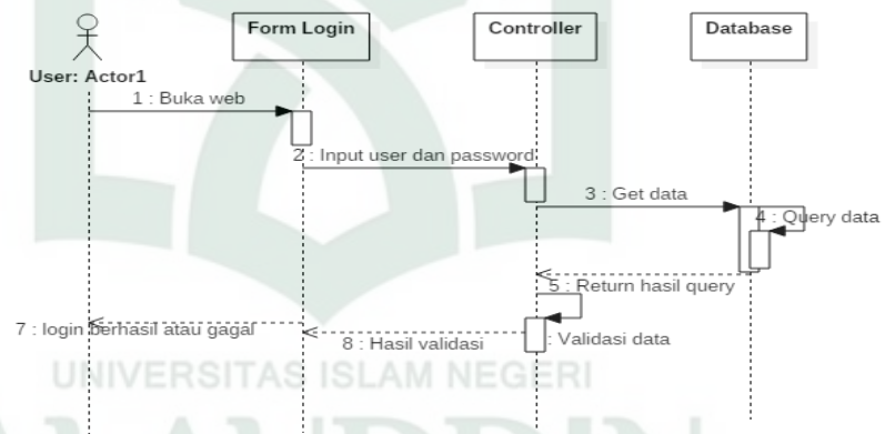
Gambar IV.15 Sequence Diagram untuk Login User
