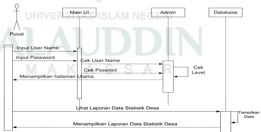
Gambar IV.17 Sequence Diagram lihat Laporan Admin
