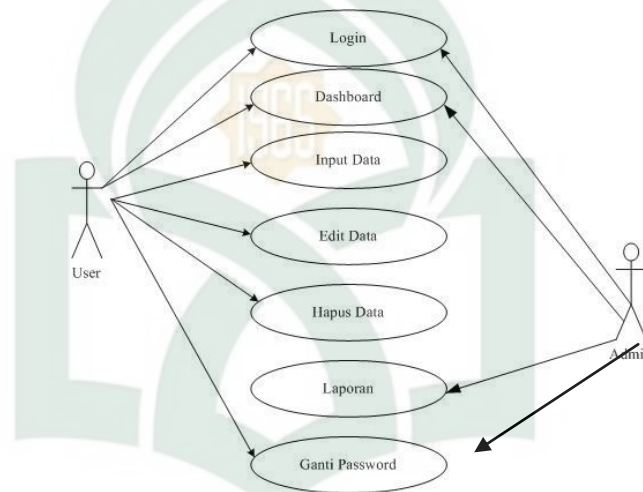
Gambar IV.3 Use Case Diagram Diusulkan
