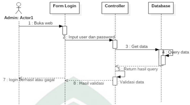
Gambar IV.14 Sequence Diagram untuk Login Admin
