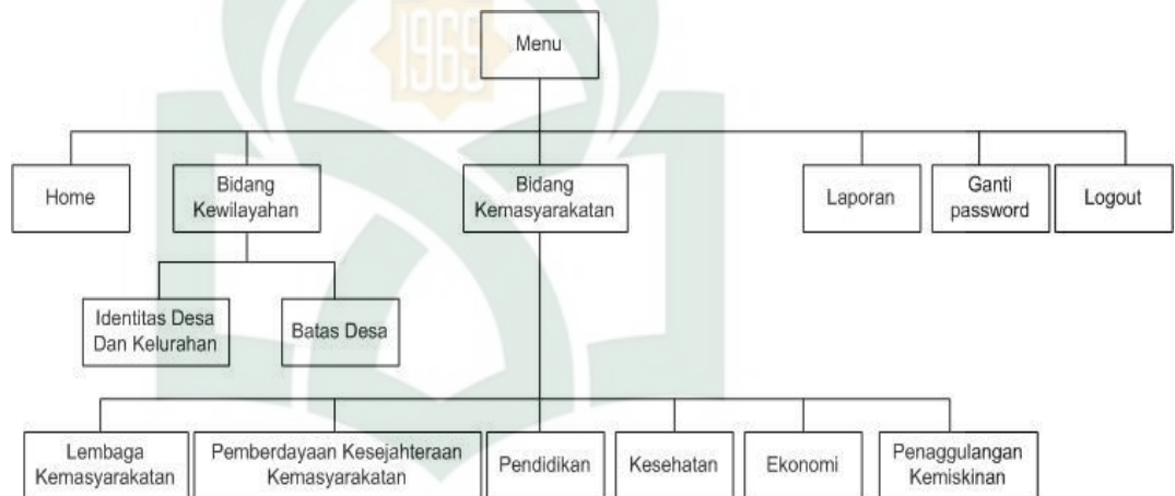
Gambar IV.18 Struktur Navigasi
