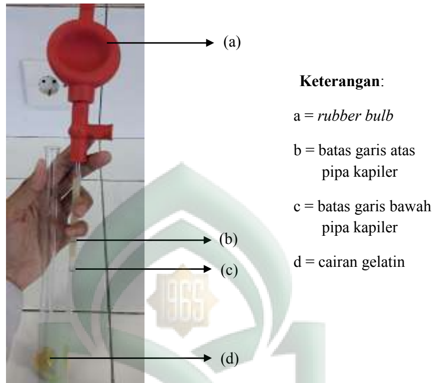
Gambar 42. Pengukuran viskositas dengan menggunakan alat viskometer ostwald
