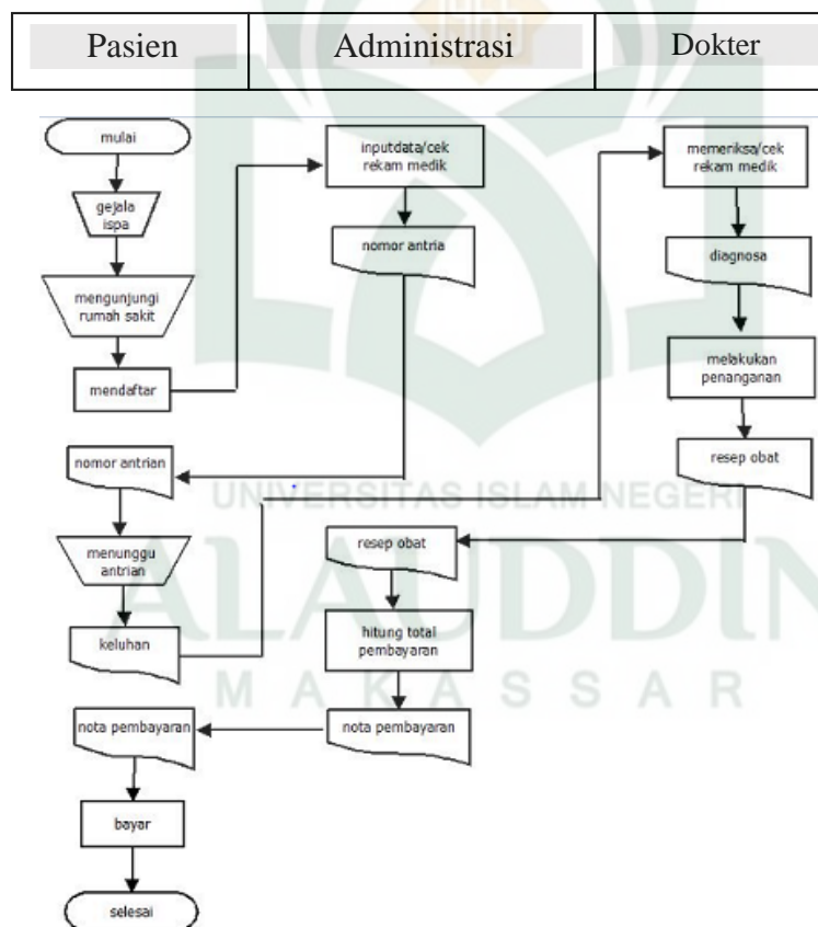
Gambar IV-1. Flowmap Pada Sistem Yang Sedang Berjalan
