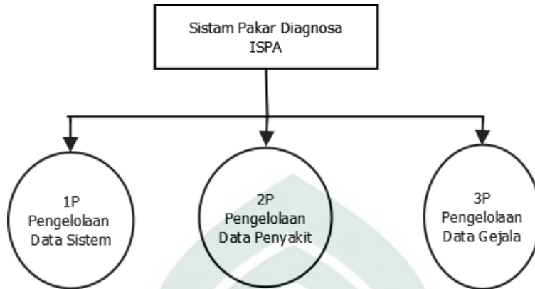
Gambar IV-3. Diagram Berjenjang
