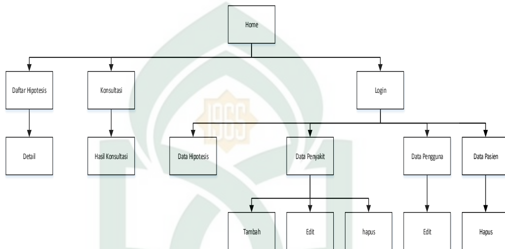
Gambar IV-10. Struktur Navigasi
