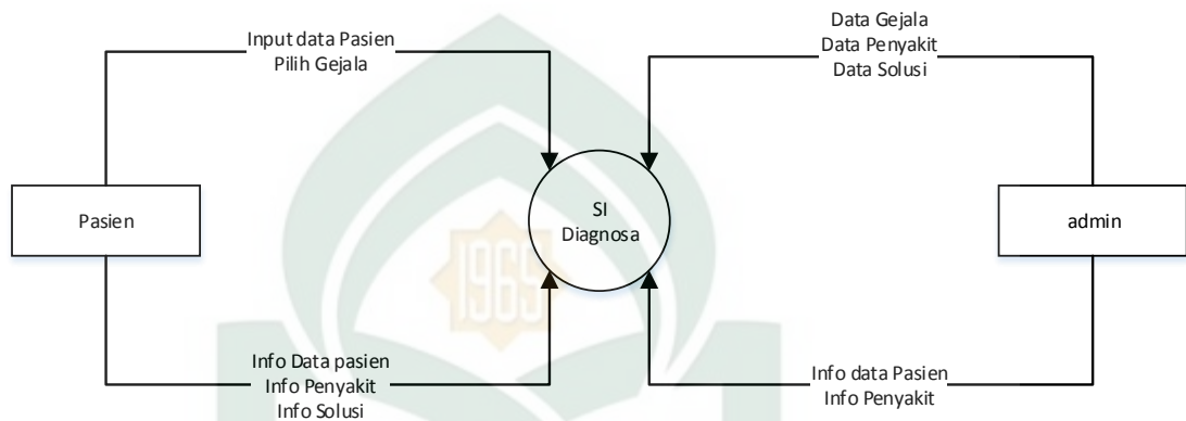
Gambar IV-5. Diagram Konteks
