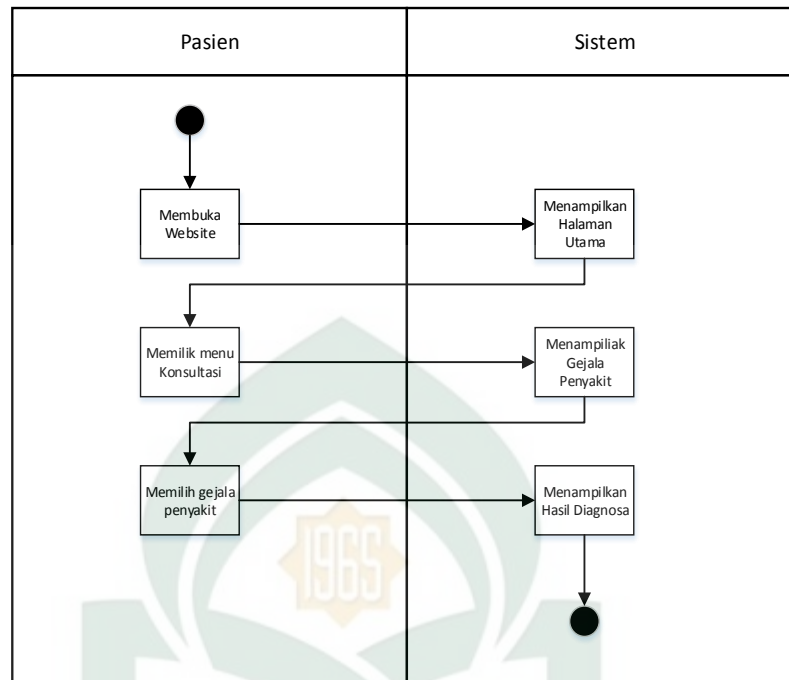
Gambar IV-6. Activity Diagram Aplikasi
