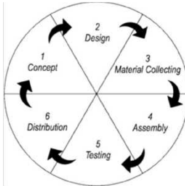
Gambar III. 1. Metode Pengembangan
