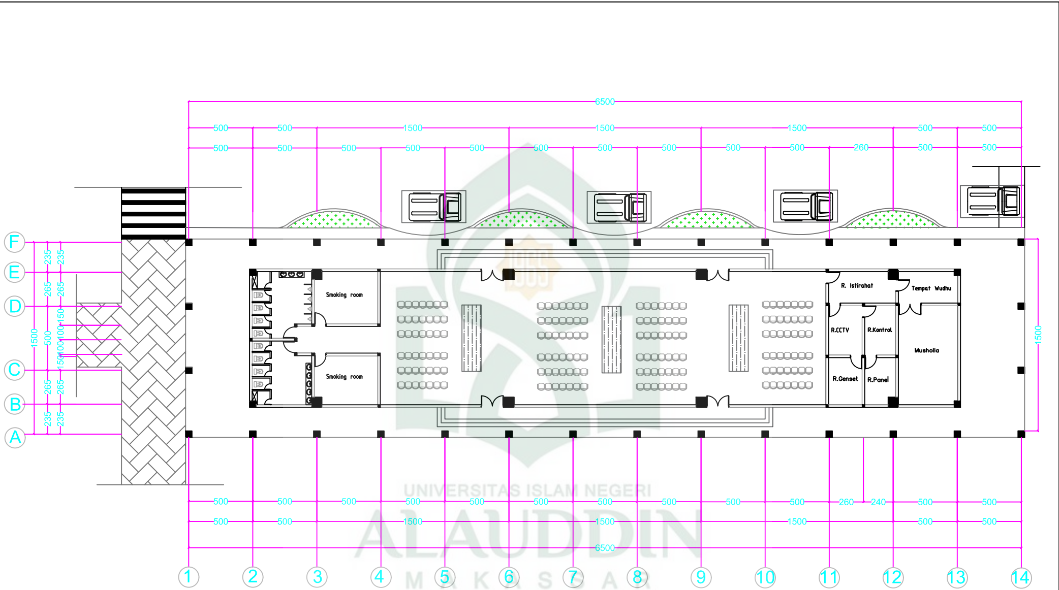
05 DENAH RG.TUNGGU PENUMPANG PETE - PETE SKALA = 1:300
