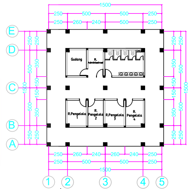
04 DENAH RG. PENGELOLA TPR SKALA = 1:300
