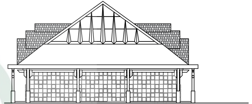
TAMPAK S. KANAN (C) SKALA = 1:300
