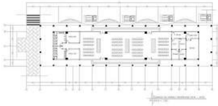
Gambar VI.3 Denah Ruang Tunggu Pete-Pete (Sumber : Hasil Desain, 2018)
