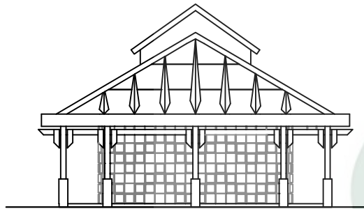
TAMPAK DEPAN (H) SKALA = 1:300
