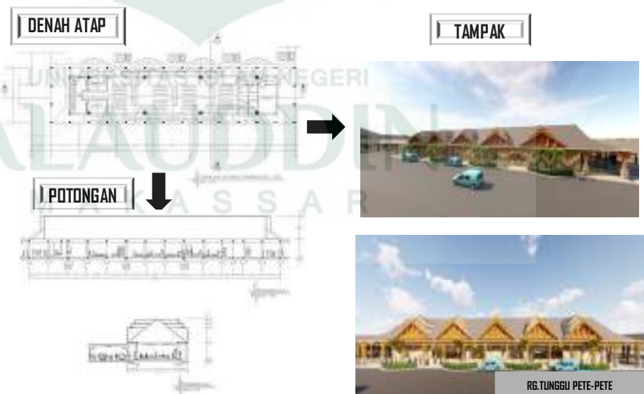
Gambar VI.12 Ruang Tunggu Pete-Pete (Sumber : Hasil Desain, 2018)
