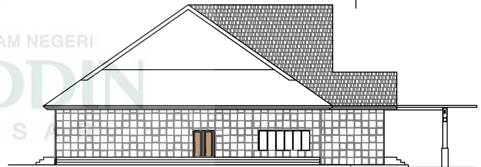
TAMPAK S. KIRI (C) SKALA = 1:300
