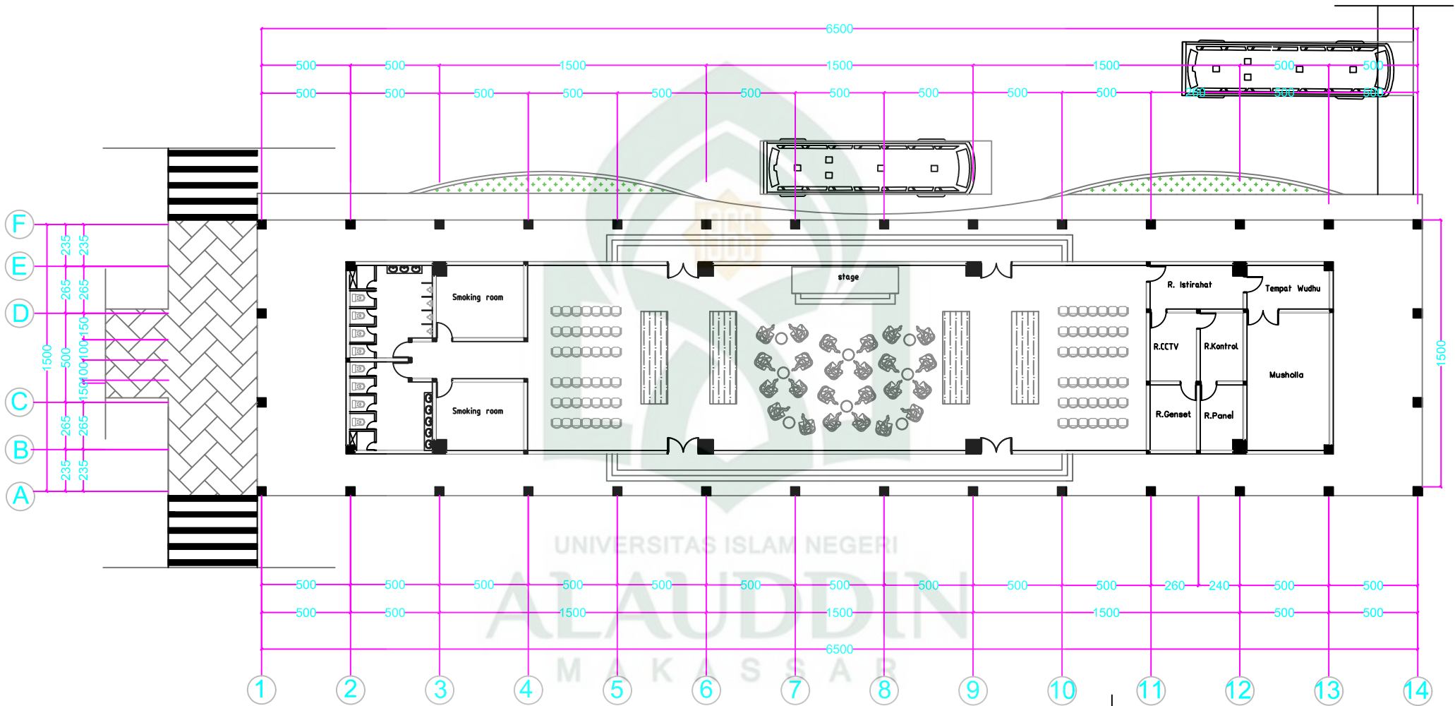
07 DENAH RG.TUNGGU PENUMPANG BUS SKALA = 1:300
