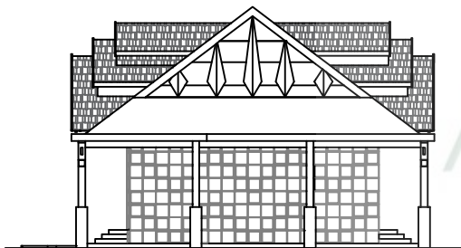
TAMPAK S. KANAN (G) SKALA = 1:300
