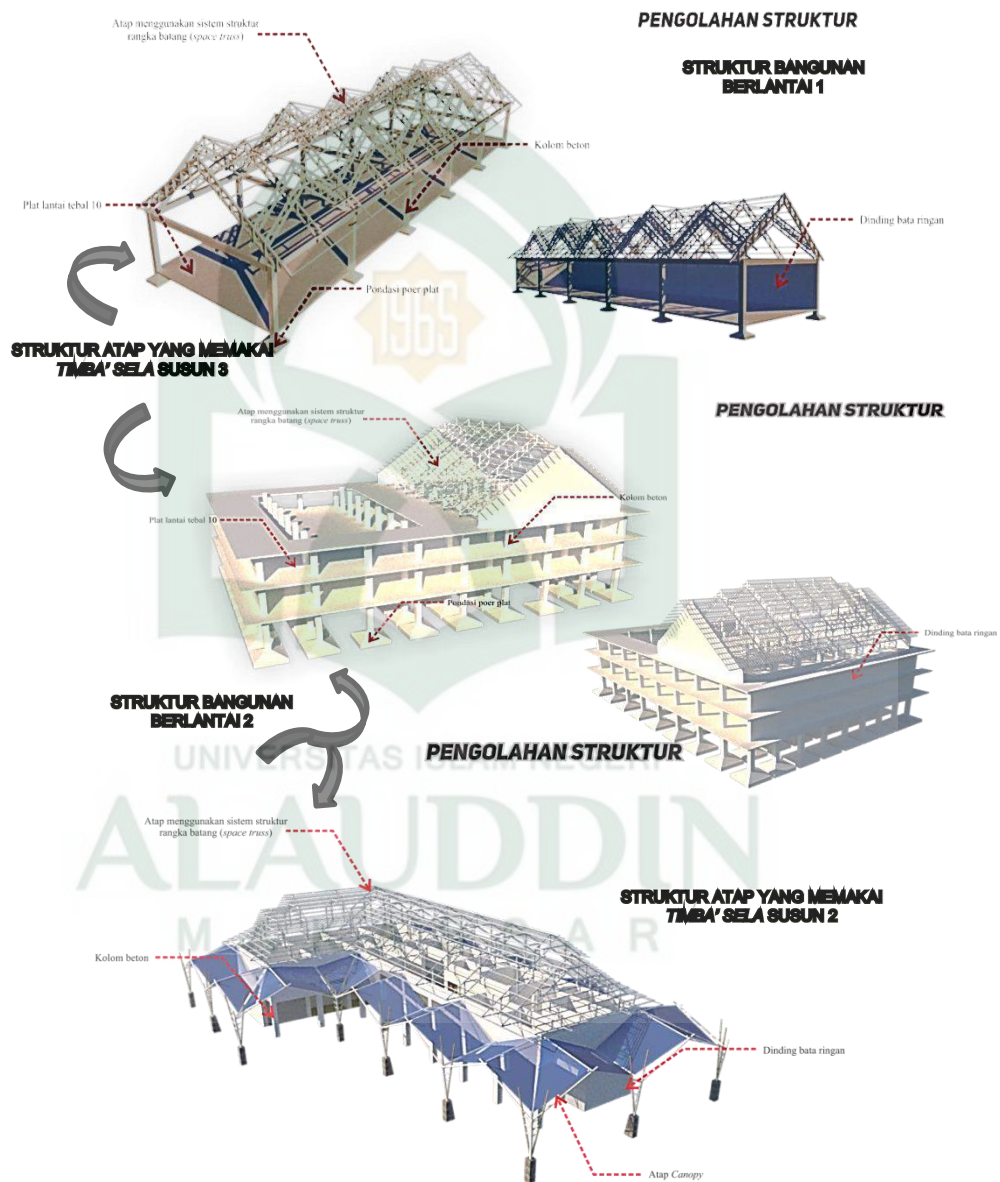
Gambar V.4 Transformasi Struktur (Sumber : Hasil Desain, 2018)
