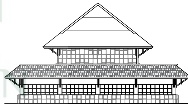
TAMPAK S. KIRI (I) SKALA = 1:300
