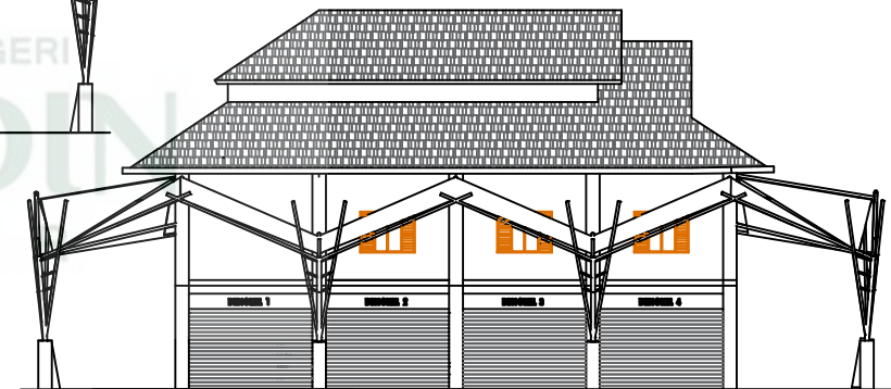
TAMPAK S. KIRI (J) SKALA = 1:300
