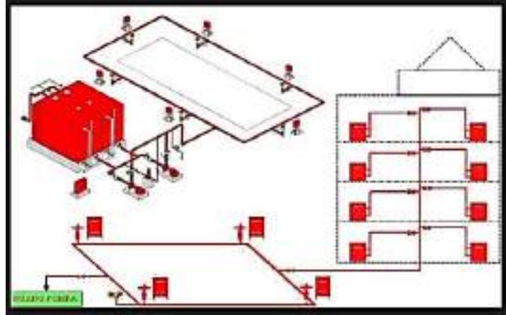
Gambar III.38 Sistem Kerja Sprinkler dan Hydrant
