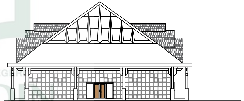
TAMPAK S. KIRI (C) SKALA = 1:300
