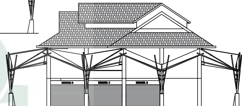
TAMPAK S. KANAN (J) SKALA = 1:300
