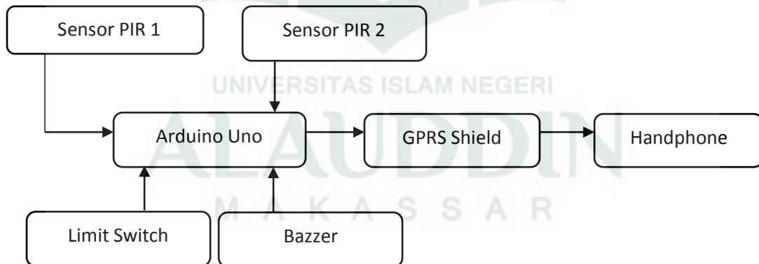
Gambar : IV.12. Blok Diagram Sistem
