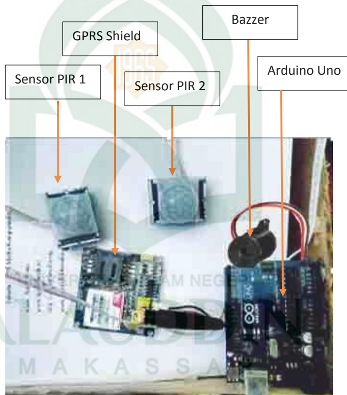
Gambar : V.18. Hasil Rancangan Perangkat Keras Dari Alat Pengaman Rumah
