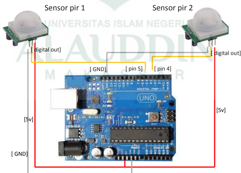
Gambar : IV.13. Konfigurasi Sensor PIR Ke Arduino Uno
