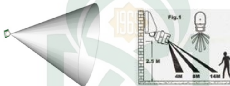
Gambar : II.7. Jarak Pancaran Sensor PIR
