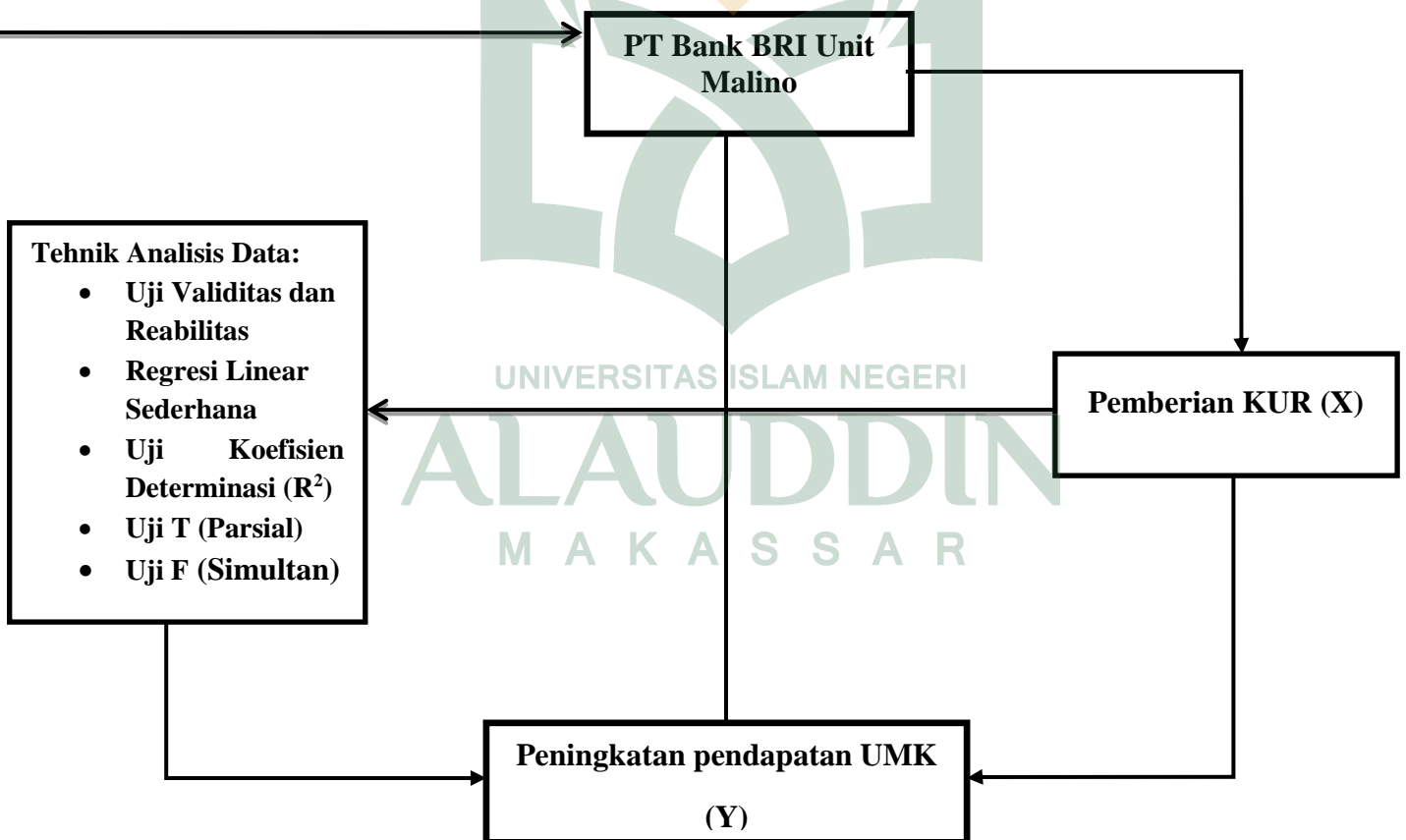
Gambar 2.1 Kerangka Pikir
