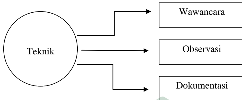
Gambar 1 Triangulasi Teknik
