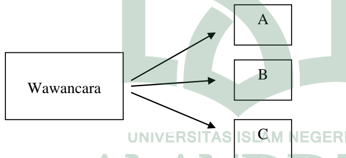
Gambar 2 Triangulasi Sumber
