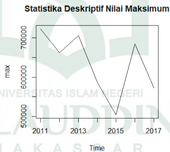
Gambar 4.3 Plot Data Statistik Deskriptif Nilai Maksimum 2011-2017
