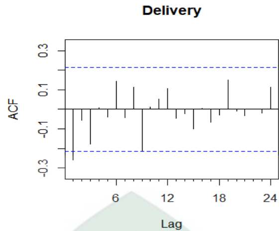
Gambar 4.6 Plot Fungsi Autokorelasi Data Jumlah Permintaan Gula Rafinasi Periode 2011-2017 Hasil Differencing Pertama
