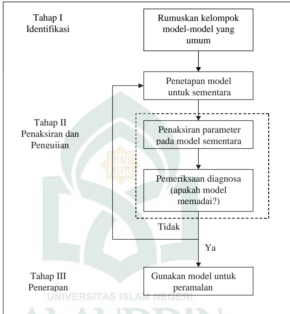
Gambar 2.1 Skema pendekatan Box-Jenkins
