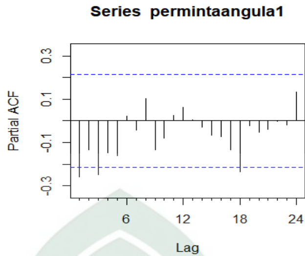
Gambar 4.7 Plot Fungsi Autokorelasi Parsial Data Jumlah Permintaan Gula Rafinasi Periode 2011-2017 Hasil Differencing Pertama
