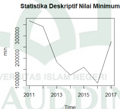
Gambar 4.1 Plot Data Statistik Deskriptif Nilai Minimum 2011-2017
