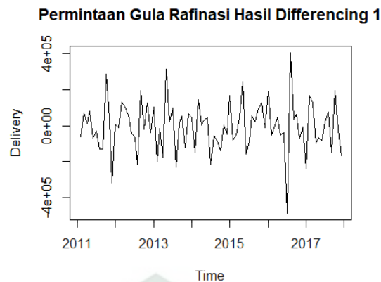
Gambar 4.5 Plot Data Jumlah Permintaan Gula Rafinasi Periode 2011-2017 Hasil Differencing Pertama
