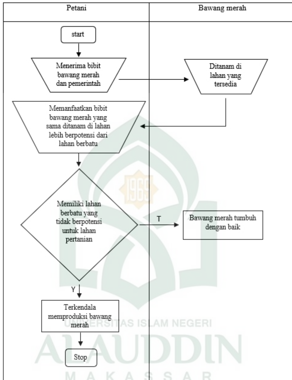
Gambar IV.4 flowmap sistem yang sedang berjalan
