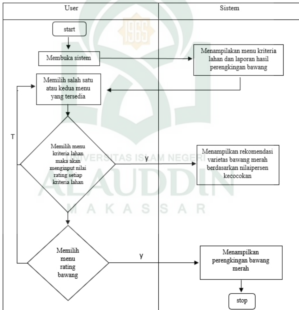
Gambar IV.5 flowmap sistem yang diusulkan
