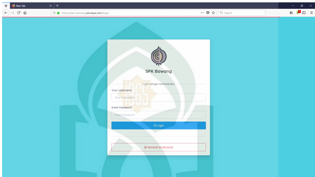
Gambar V.24 Antarmuka Login
