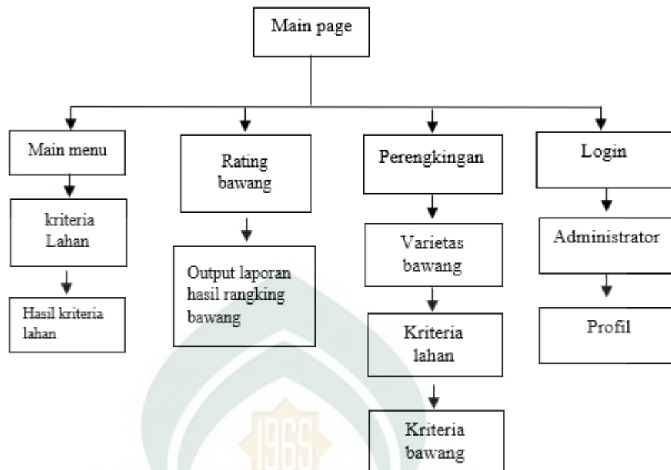
Gambar IV.11 Struktur navigasi
