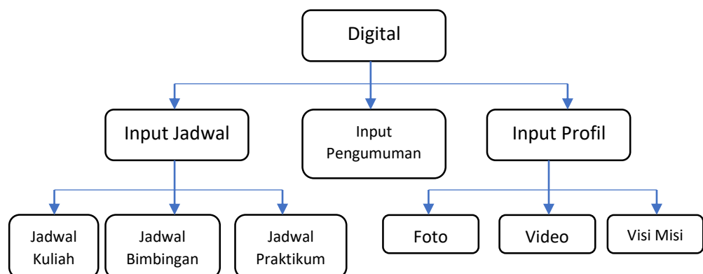
Gambar IV.6 Diagram Berjenjang
