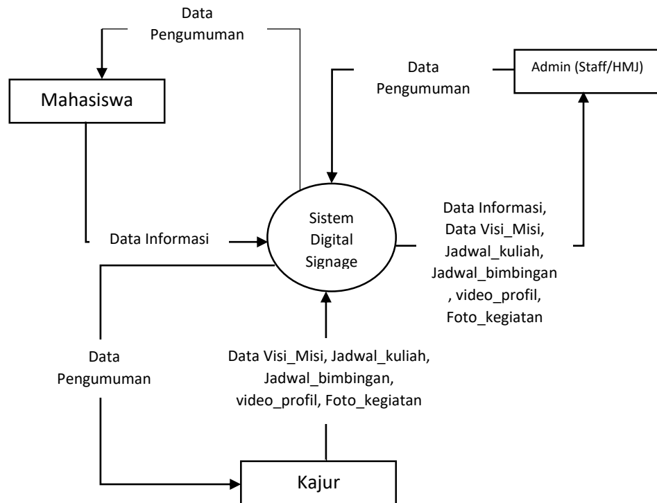
Gambar IV.5 Diagram Konteks
