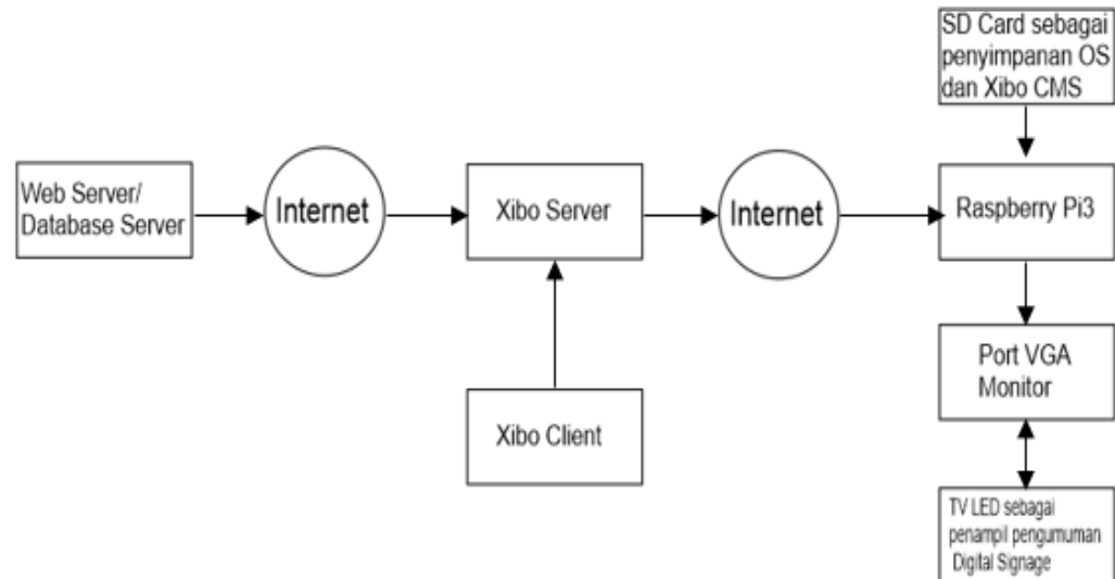
Gambar IV.3 Diagram Blok Raspberry Pi3 pada sistem
