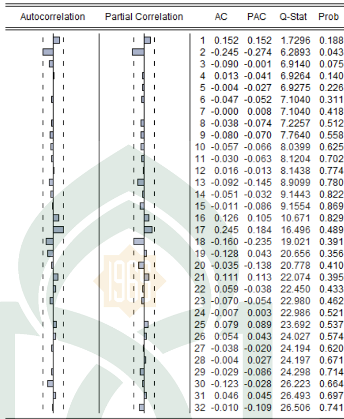
Gambar 4.31: collogram dari data inflasi kelompok transportasi
