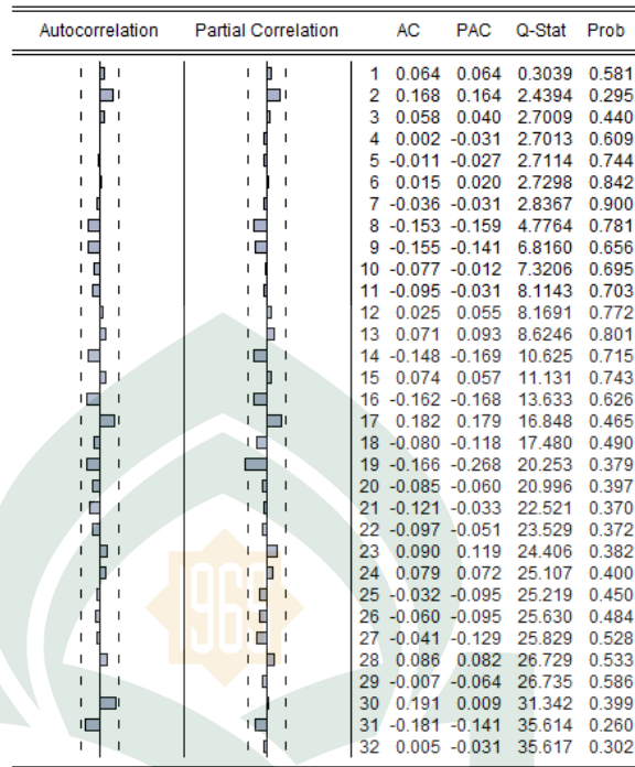
Gambar 4.11: collegram dari data inflasi kelompok perumahan
