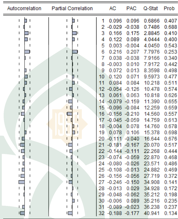
Gambar 4.21: collegram dari data inflasi kelompok kesehatan
