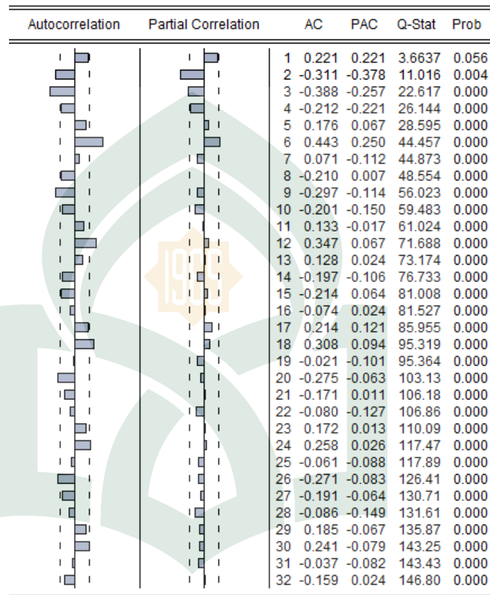
Gambar 4.1: collegram dari data inflasi kelompok bahan makanan
