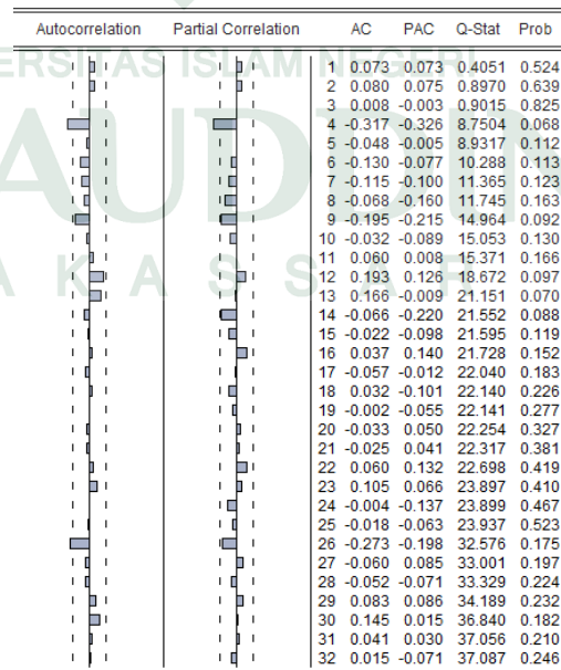
Gambar 4.16: collogram dari data inflasi kelompok sandang
