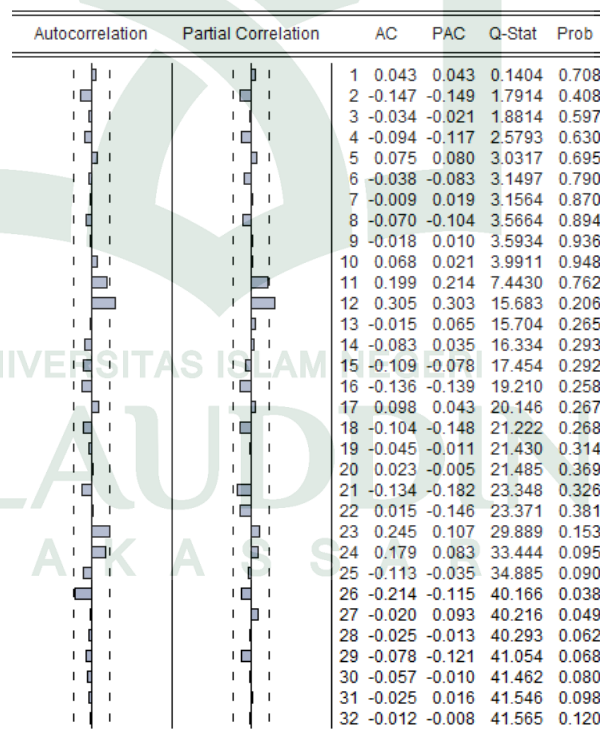
Gambar 4.6: collegram dari data inflasi kelompok makanan jadi
