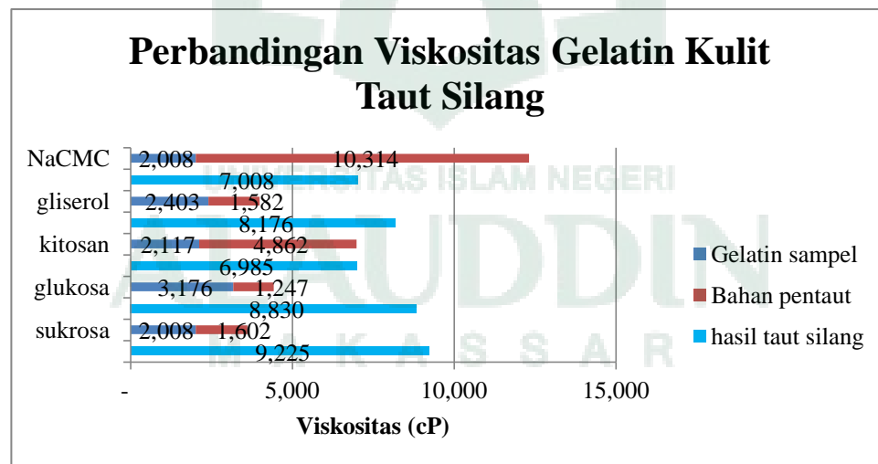
Gambar 17. Hasil perbandingan peningkatan viskositas gelatin kulit sapi taut silang.
