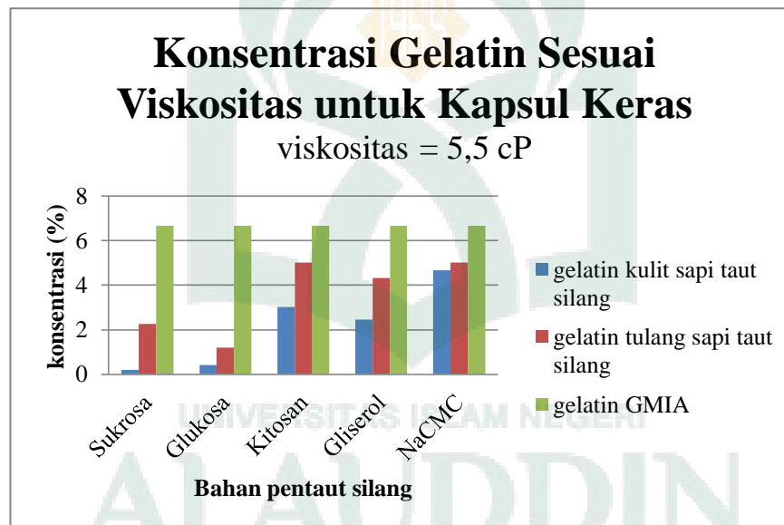
Gambar 21. Hasil perhitungan kebutuhan konsentrasi gelatin untuk kapsul keras
