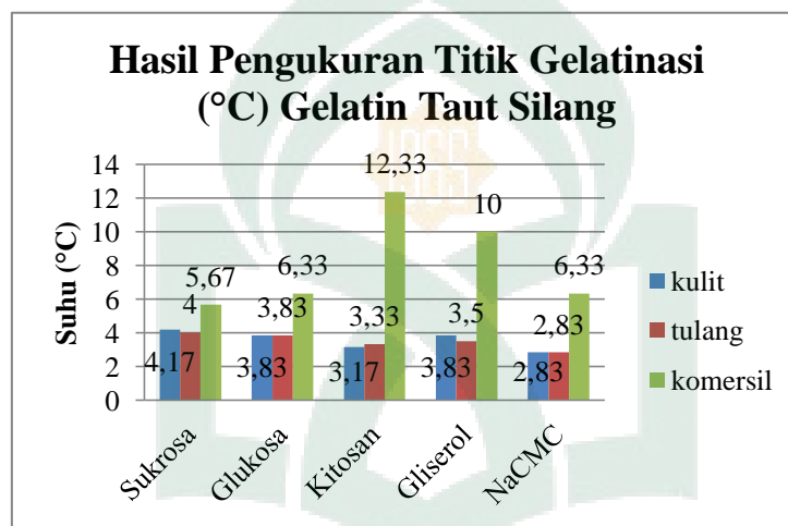
Gambar 15. Hasil pengukuran titik gelatinasi gelatin taut silang
