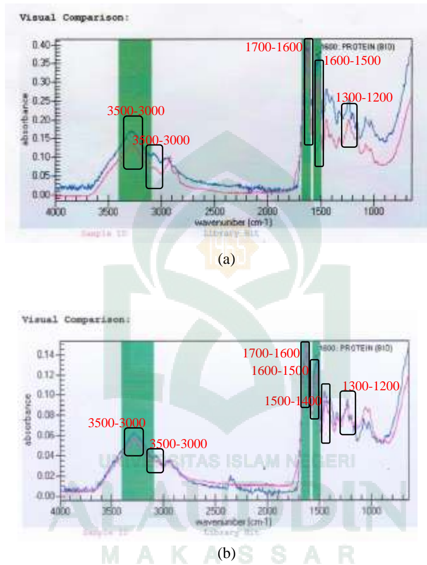
Gambar 5. hasil pengukuran FTIR gelatin (a) kulit sapi, (b) kulit sapi + NaCMC.
