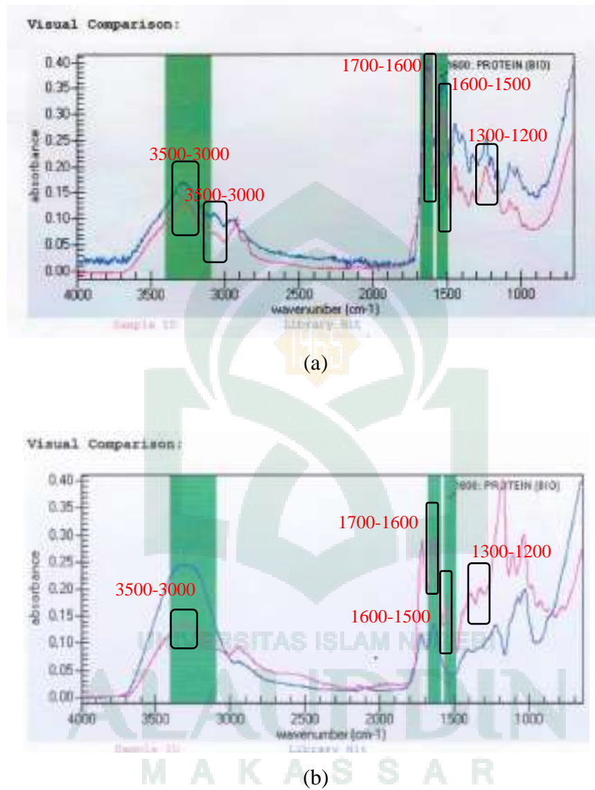
Gambar 4. hasil pengukuran FTIR gelatin (a) kulit sapi, (b) kulit sapi + gliserol.
