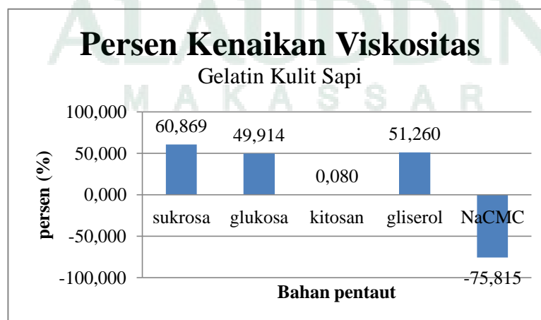
Gambar 19. Persen Peningkatan Viskositas Gelatin Kulit Sapi Taut Silang
