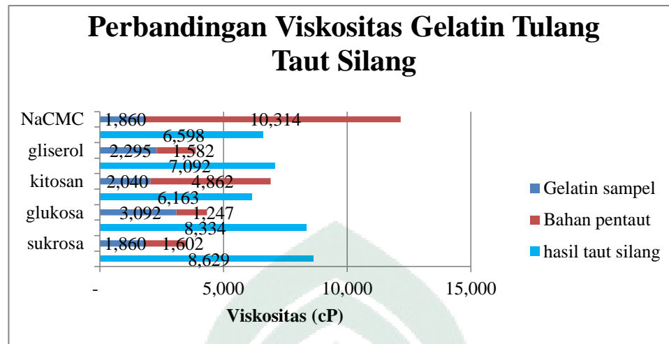
Gambar 18. Hasil perbandingan peningkatan viskositas gelatin kulit sapi taut silang.
