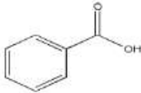
Gambar 7. Rumus Struktur Natrium Benzoat
