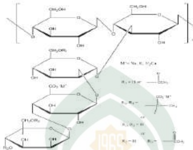
Gambar 6. Rumus Struktur Xantan Gum
