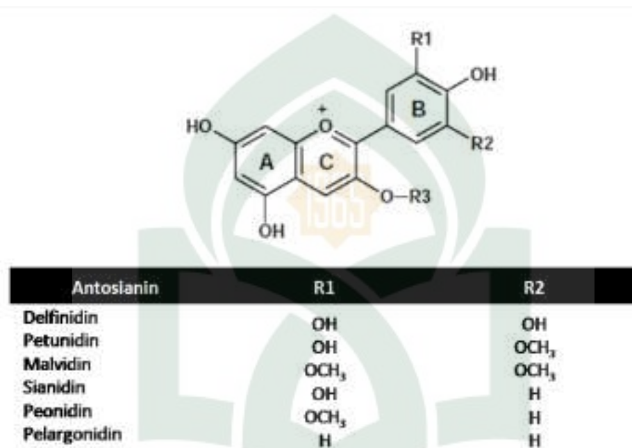
Gambar 2. Rumus Struktur Antosianin
