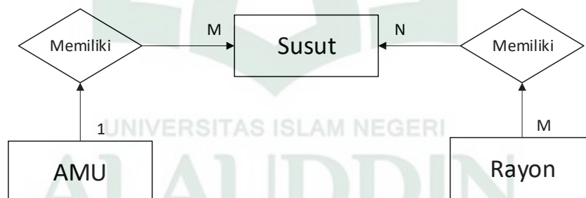
Gambar IV.6. ERD Sistem
