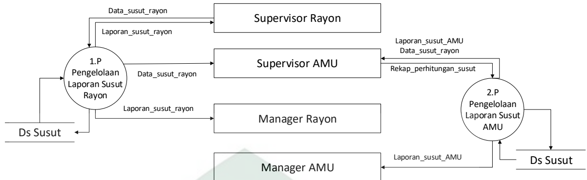
Gambar IV.5. DFD Level 1
