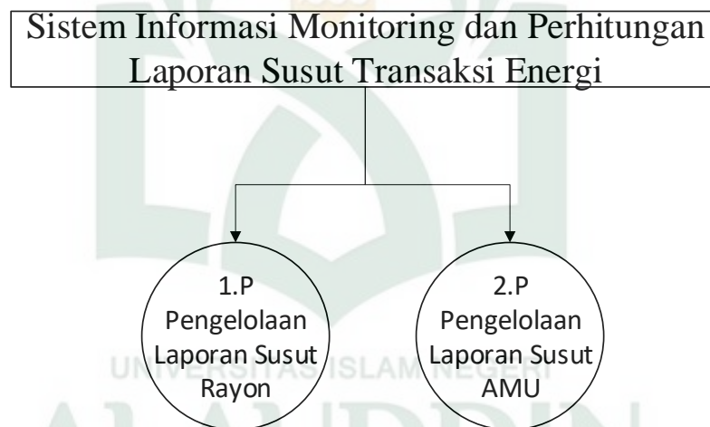
Gambar IV.4. Diagram Berjenjang
