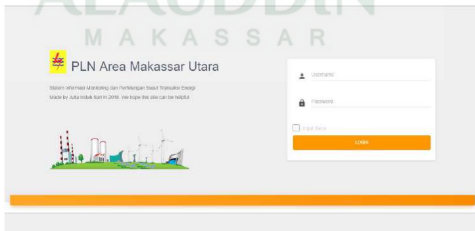
Gambar V.1 Antarmuka Login
