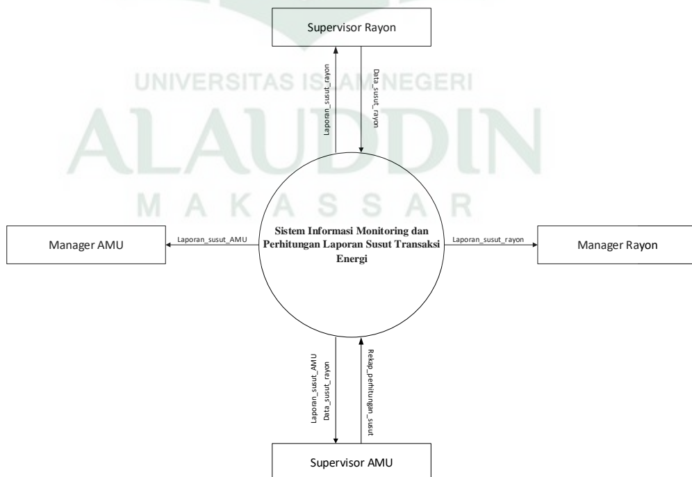
Gambar IV.3. Diagram konteks
