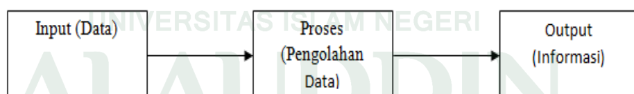
Gambar 1.1. Siklus Informasi
