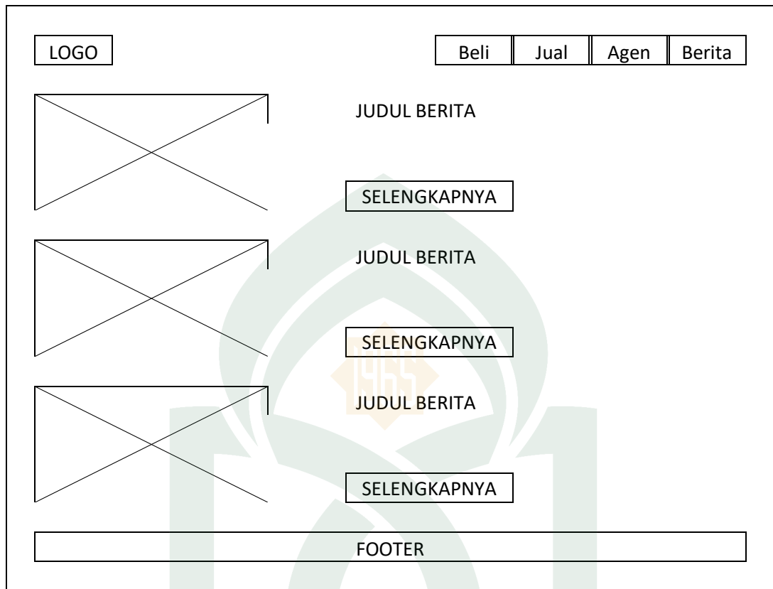
Gambar IV.19. Halaman Berita
