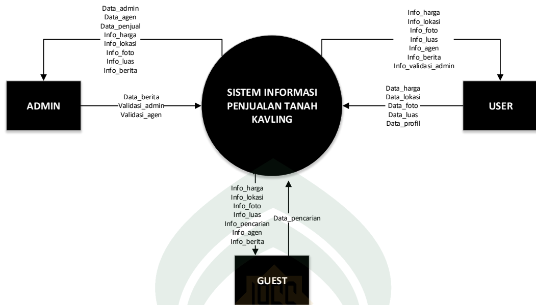
Gambar IV.5. Diagram konteks
