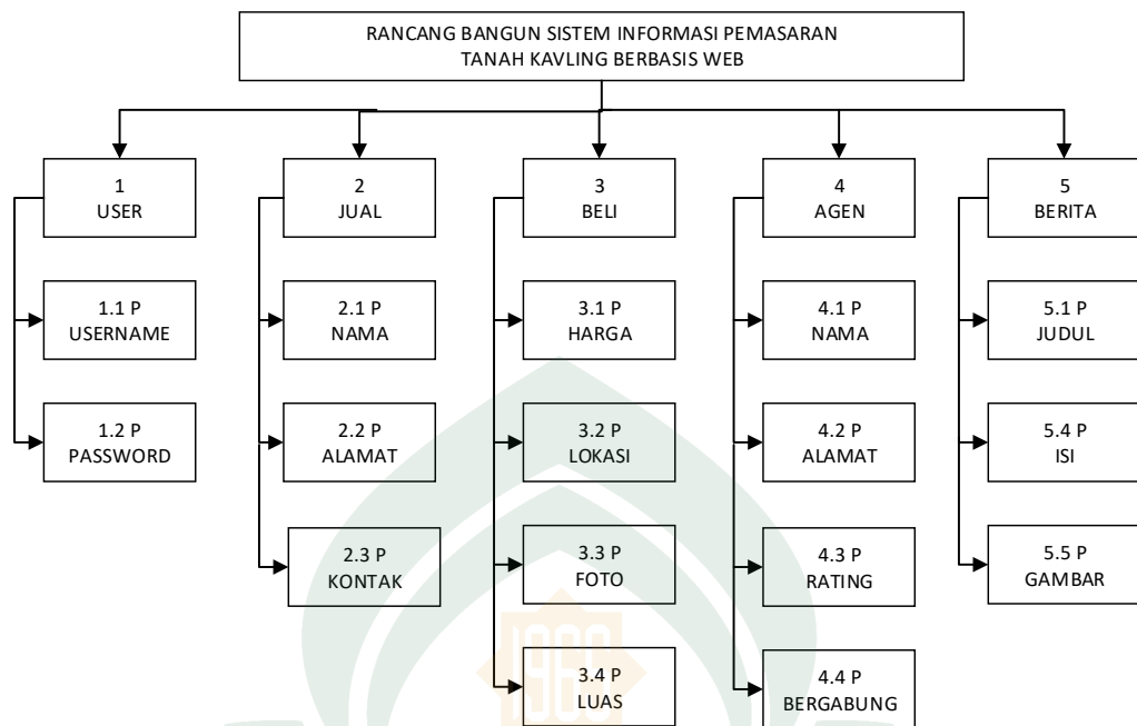
Gambar IV.4. Diagram berjenjang
