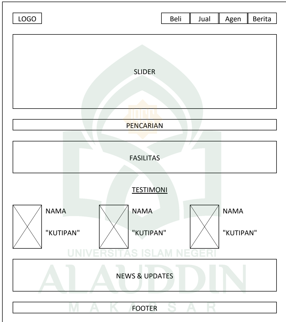
Gambar IV.14. Halaman Beranda
