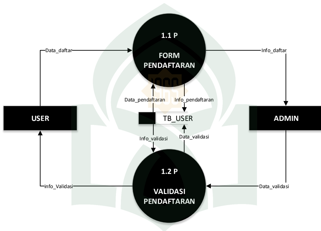
Gambar IV.7. DFD level 2 proses 1
