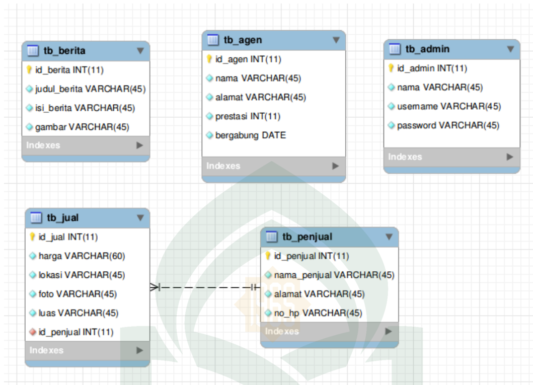
Gambar IV.13. Desain Tabel Sistem
