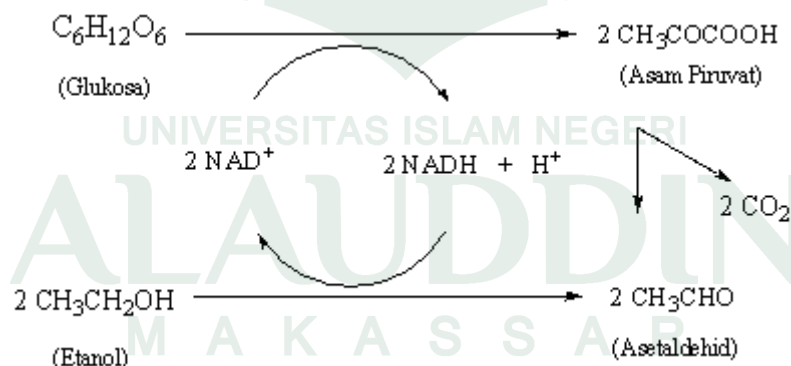
Gambar 4.5 Fermentasi Glukosa
